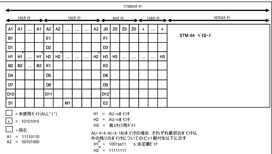
図 2-5 STM-64 信号のフレームフォーマット
