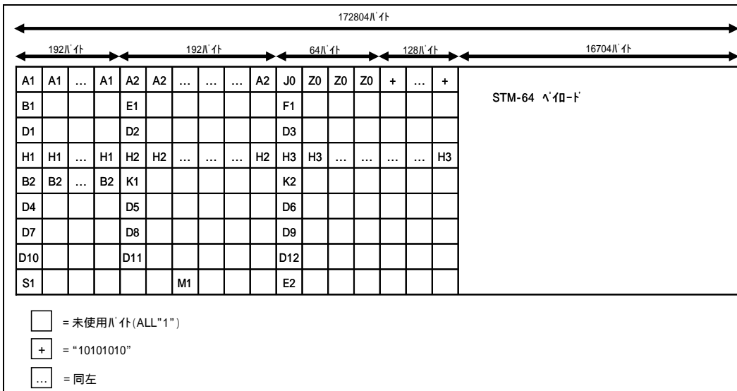
図 2-5 STM-64 信号のフレームフォーマット
