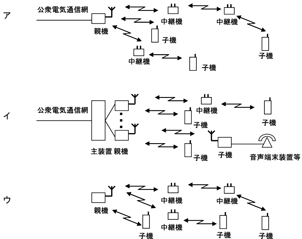
図 1. 4-7 DECT 準拠方式のシステム構成例
