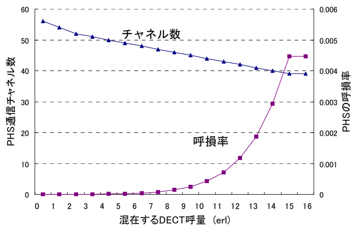
図 3. 2-14 DECT 準拠方式混在時における現行方式の呼損率変化
