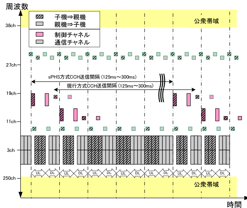
図 3. 2-8 現行方式、sPHS 方式の制御チャンネル送信
