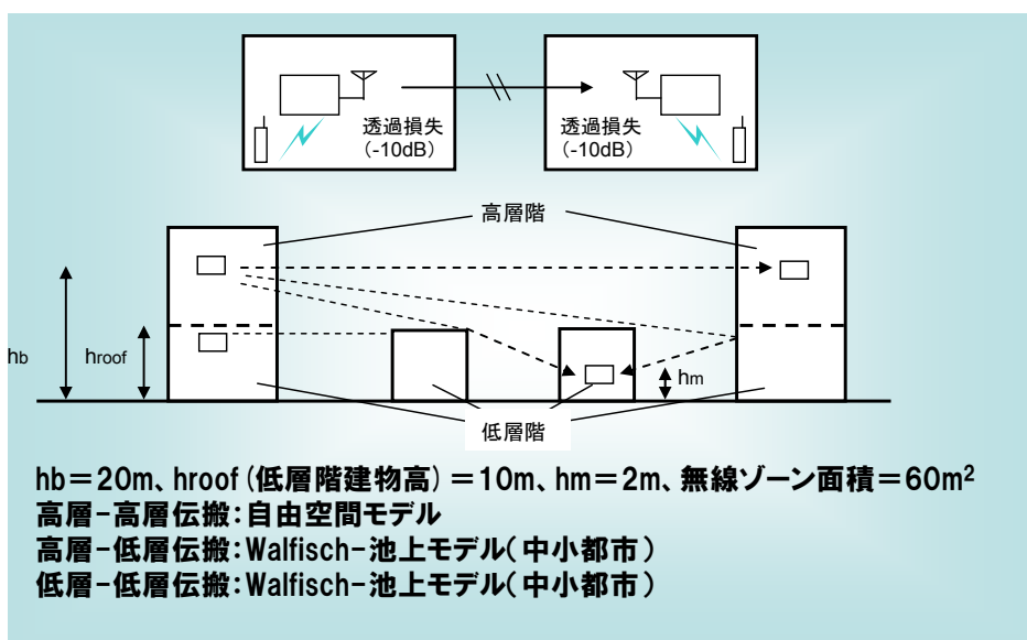
図 3. 2-12 マンション群のモデル
