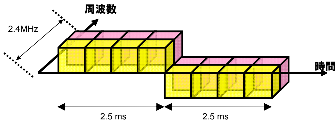
図1. 4-16 sPHS方式のフレーム構成（対称構成の場合の例）
