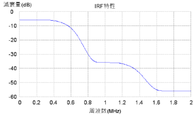
図 3. 2-5 DECT 準拠方式の IRF 特性
