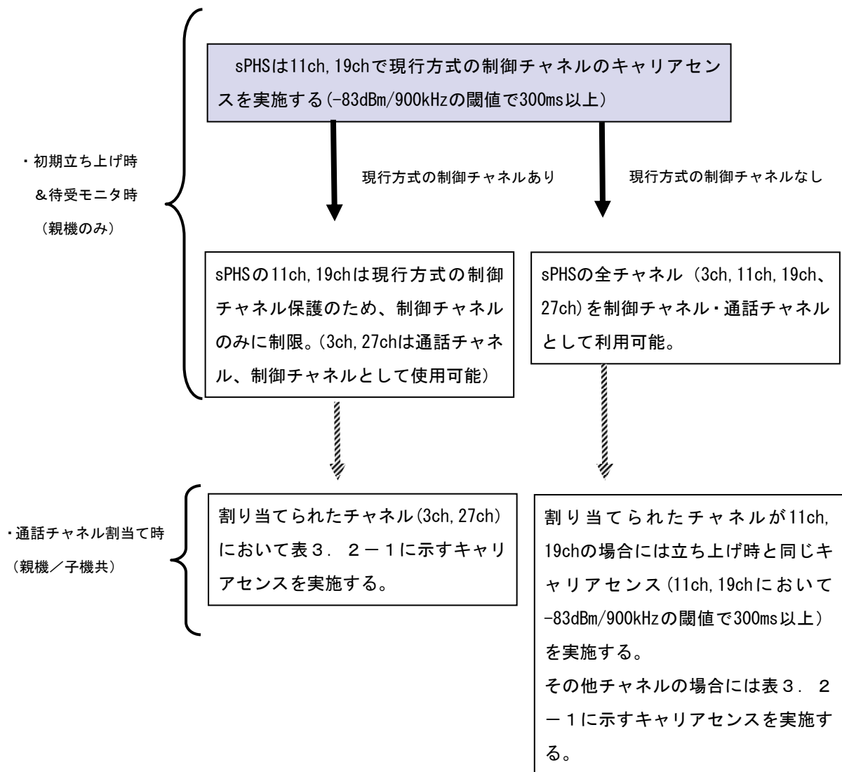
図3. 2-9 現行方式、sPHS方式の制御チャンネル送信
