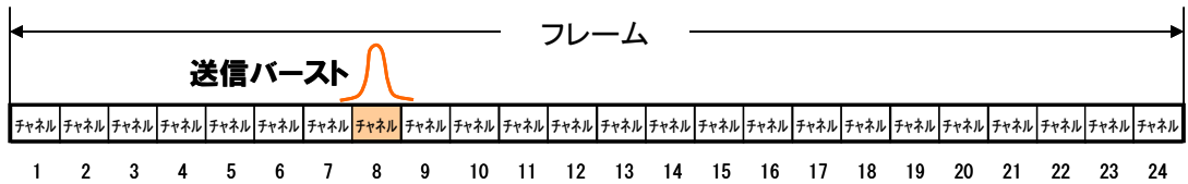
図4. 1-1 DECT 準拠方式のチャネル構成
