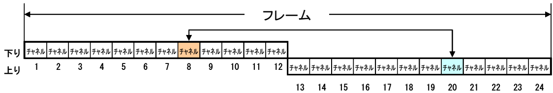
図4. 1-2 DECT 準拠方式の通話チャネル構成
