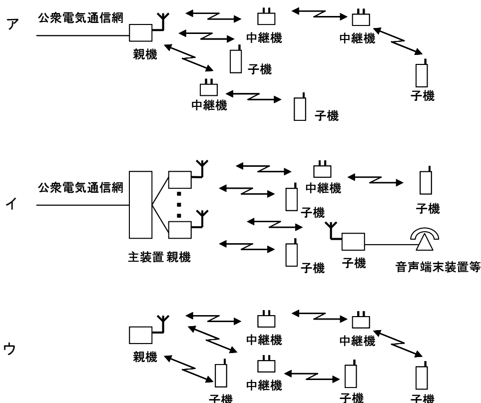
図1. 4-13 sPHS方式システム構成例
