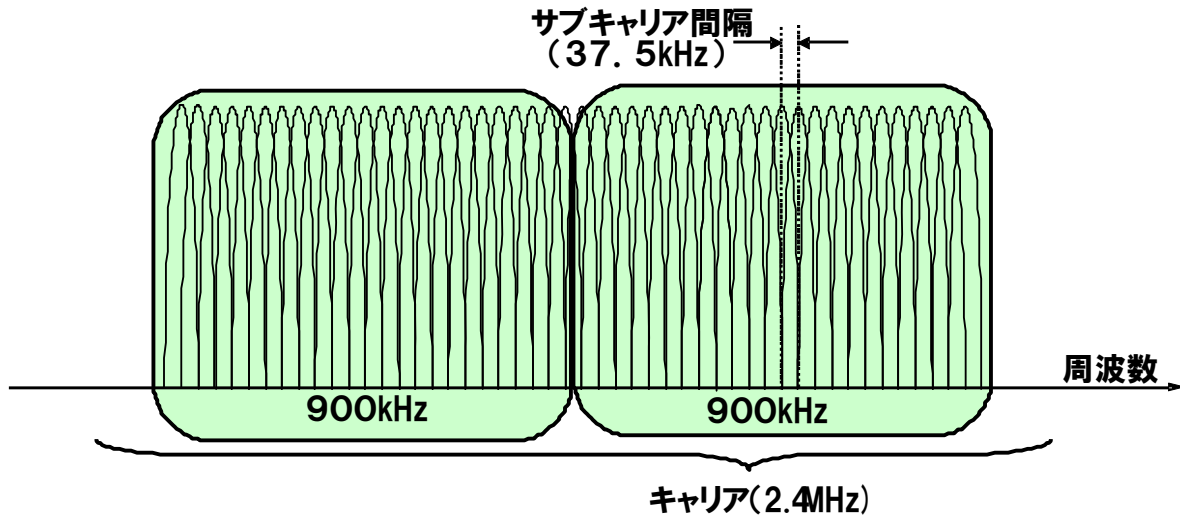
図1. 4-14 sPHS方式の周波数構成
