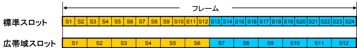
図 4. 1-3 DECT 準拠方式のスロット構成
