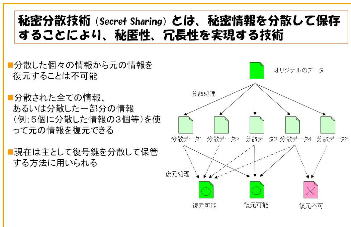
図 8 秘密分散法
