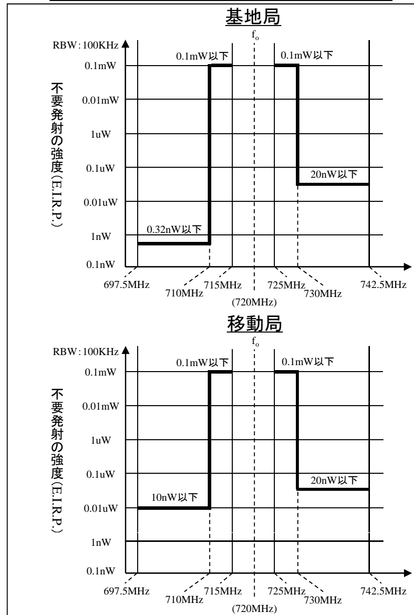
700MHzにLTE(上り)が割り当てられた場合
