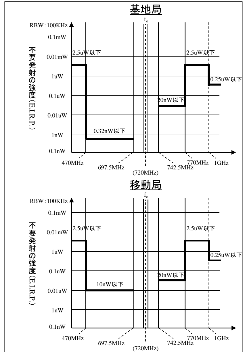
700MHzにLTE(上り)が割り当てられた場合
