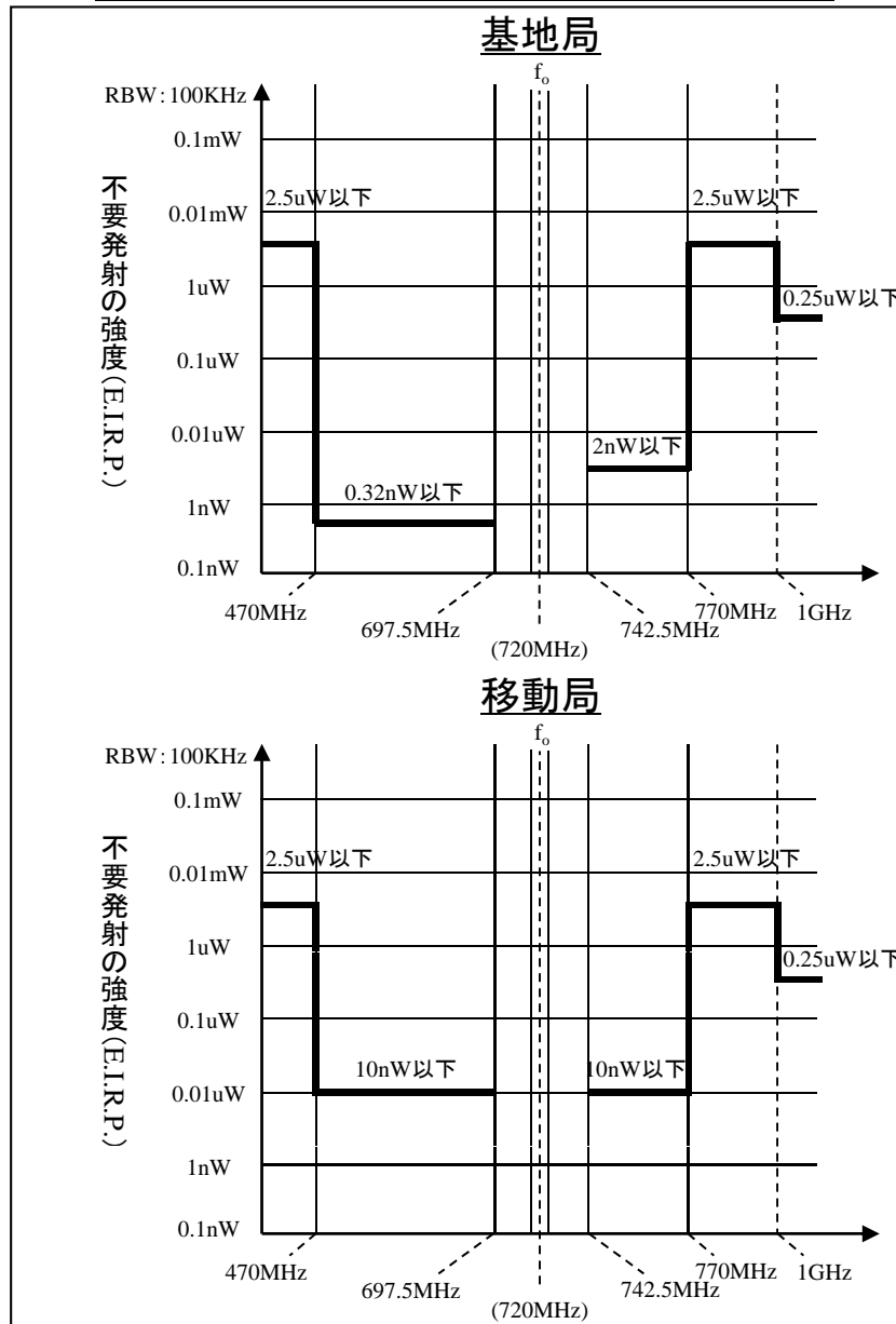
700MHzにLTE(下り)が割り当てられた場合
