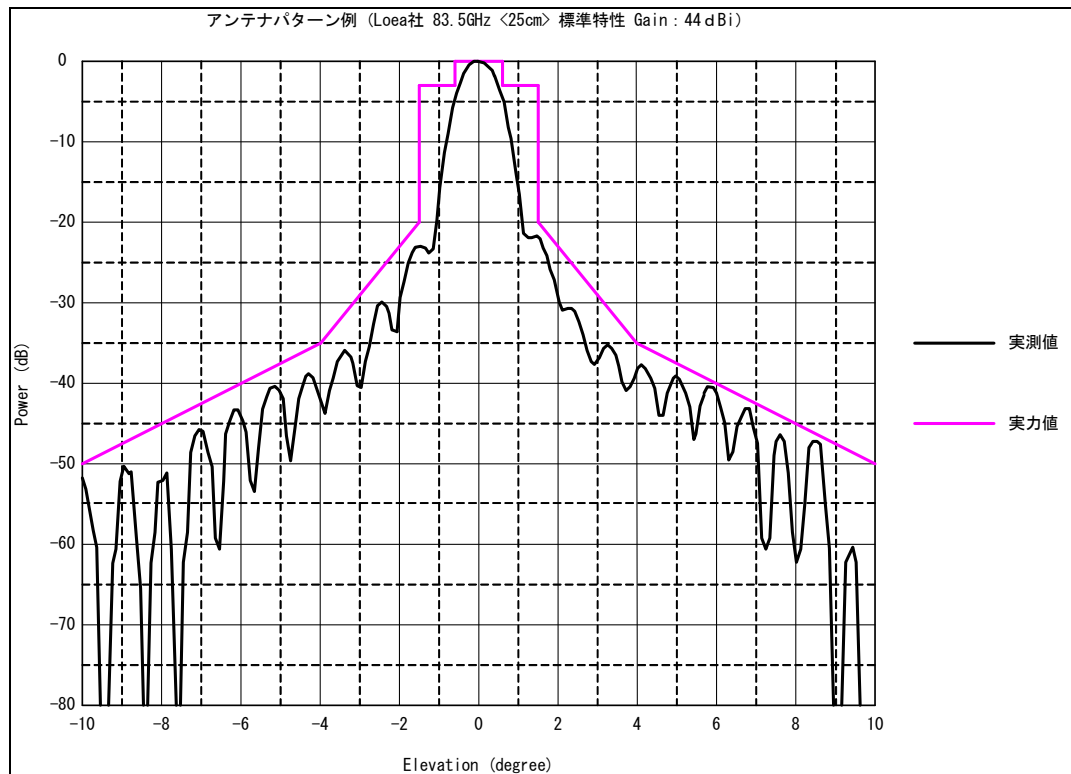
図 3-2 空中線指向特性 (口径約 25cm) の例 (利得最大点の定格約 44dBi)
