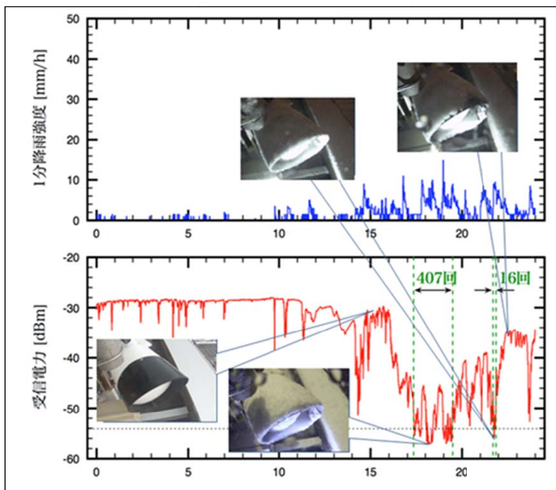
図2-2 降雪前後における通信状況の実験結果 (回数は瞬断)
