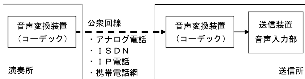
図４－２－１－７ 電話回線を利用して予備回線を構成する場合の例
