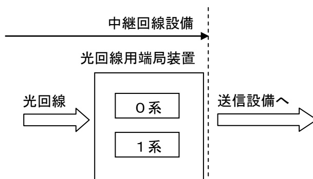
図４－２－１－５ 光回線用端局装置を二重化構成する例
