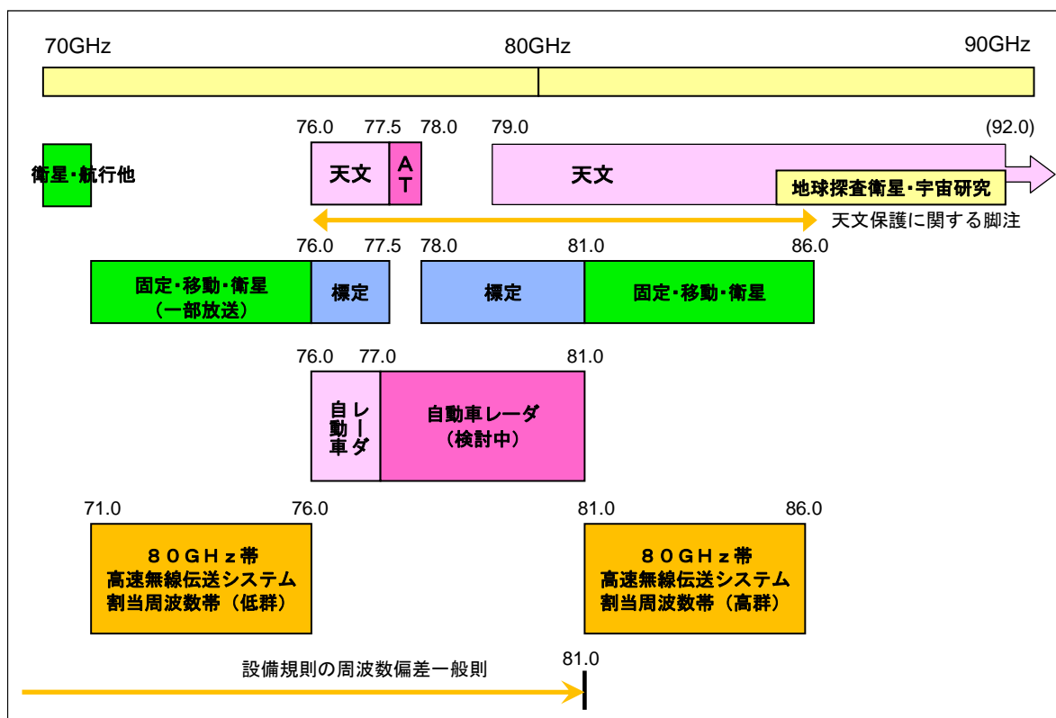
図 2 - 3 70GHz~90GHz の分配等の状況
