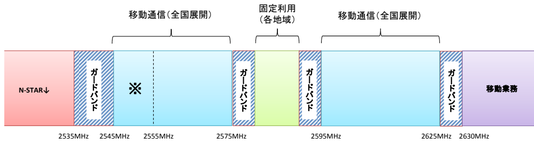
図-東-6-7 広帯域移動無線アクセスシステムの使用周波数帯
