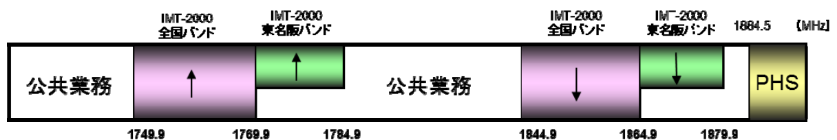
図-東-5-15 1.7GHz帯携帯無線通信用の周波数配置
