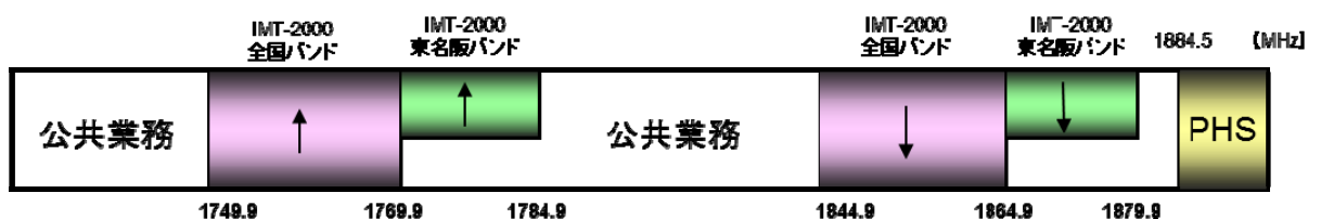
図-沖-5-12 1.7GHz帯携帯無線通信用の周波数配置
