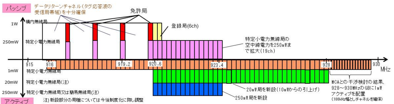
図 4-5 920MHz 帯電子タグシステム等のチャンネルプラン
