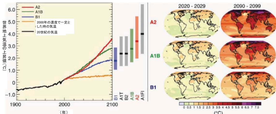
&lt;地上気温上昇(1980～1999年との比較)&gt;
