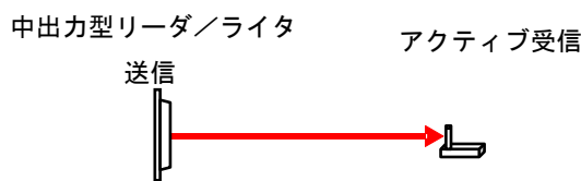
参図 7-3 中出力型 920MHz 帯パッシブタグリーダ／ライタと 920MHz 帯アクティブ系小電力システムの干渉モデル
