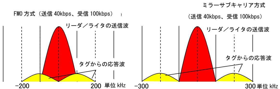
図 4-2 FMO 方式とミラーサブキャリア方式のスペクトル例
