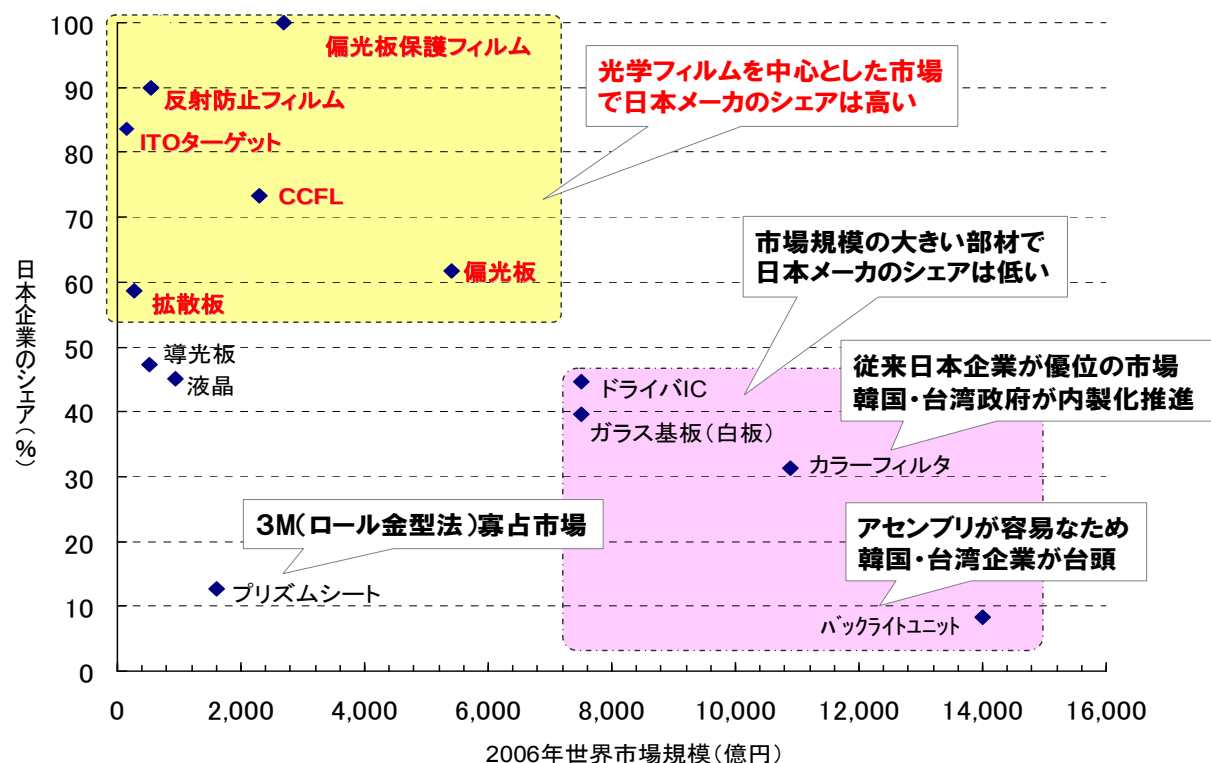
主な液晶パネル用部材の市場規模と日本企業のシェア
