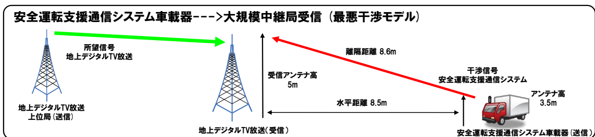
図参 7-20 モデル 5-1
