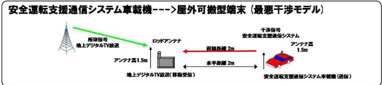
図 3.2.4-22 モデル6
