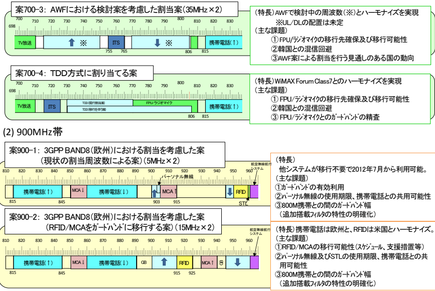
図 1.1.2-3 700/900MHz 帯割当検討モデル案
