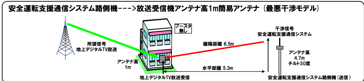
図 3.2.4-3 モデル 1-3-無
