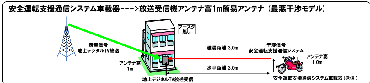
図 3.2.4-14 モデル 4-3-無
