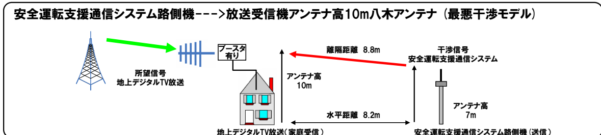
図 3.2.4-4 モデル 1-1-有
