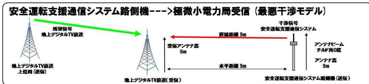
図 3.2.4-10 モデル 2-2
