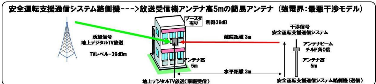
図 3.2.4-8 モデル 1-3-有
