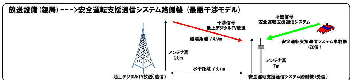
図参 7-26 モデル 8-1
