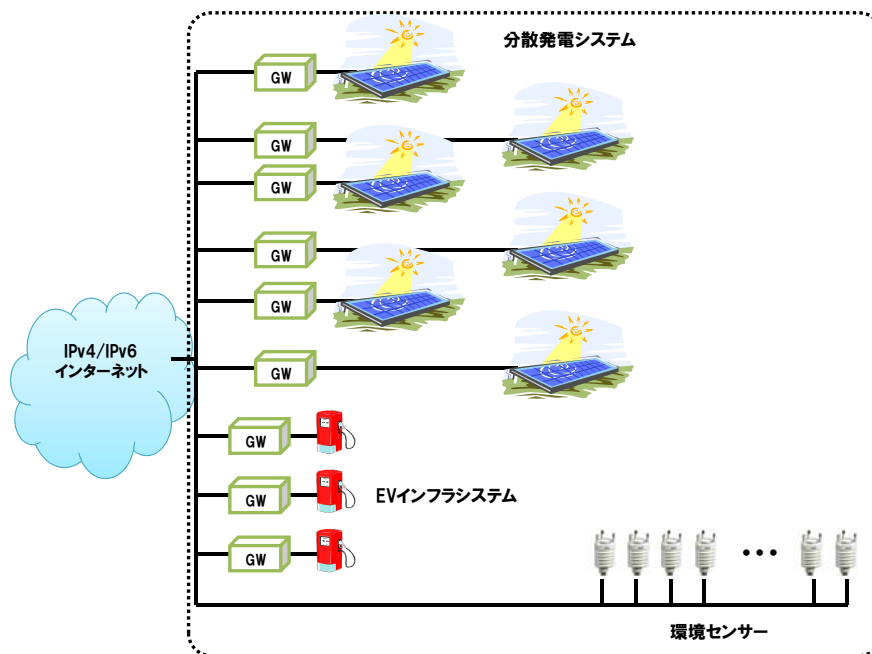
図 3-11 エネルギー情報計測・送信システムのイメージ（例）
