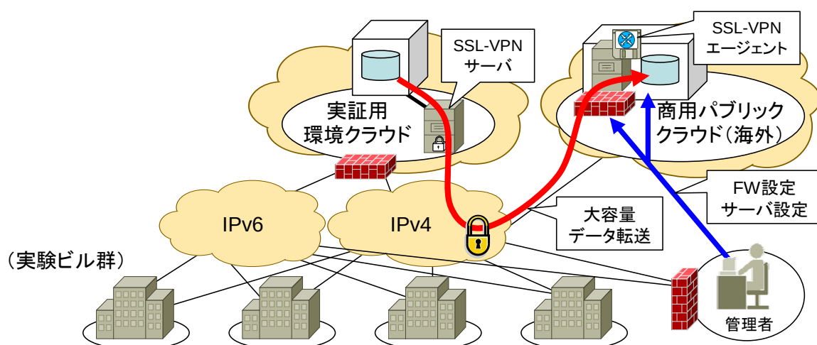
図 4-13 モデル A におけるパブリッククラウドを活用した実証
