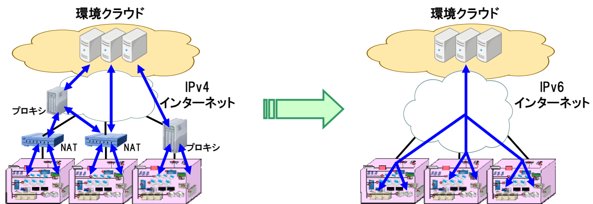
図 3-13 IPv4 と IPv6 における環境クラウドの構成
