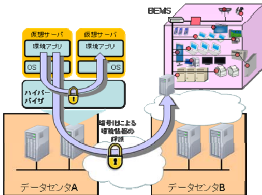
図 4-18 仮想化基盤内通信の暗号化確保の実証
