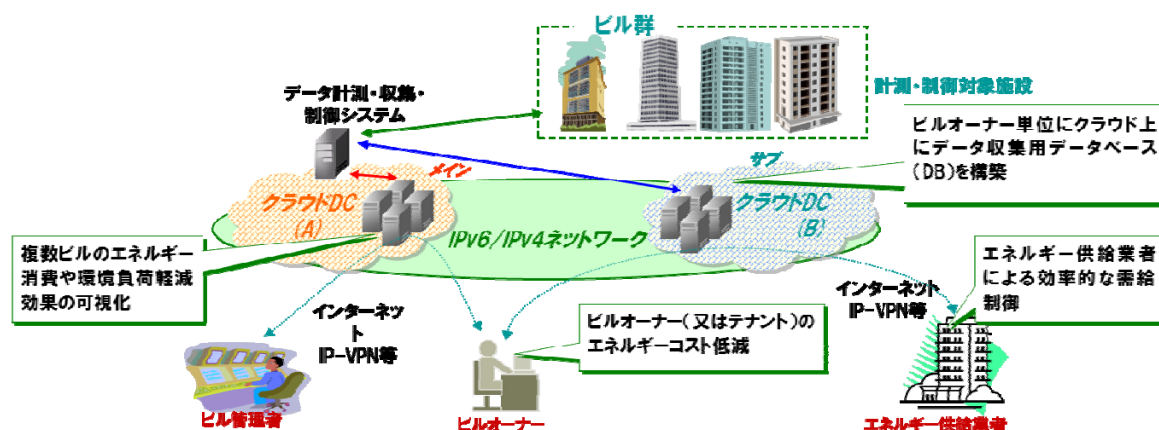
図 2-4 ビル群エネルギー管理システムにおけるデータ利用の流れ
