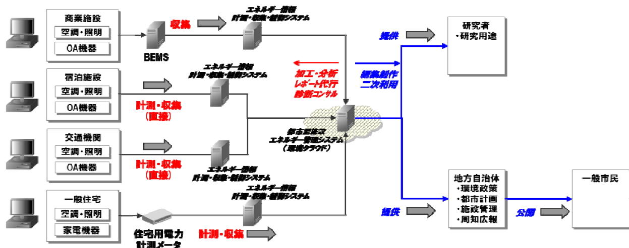
図 3-6 都市型施設エネルギー管理システムにおけるサービスモデル（例）
