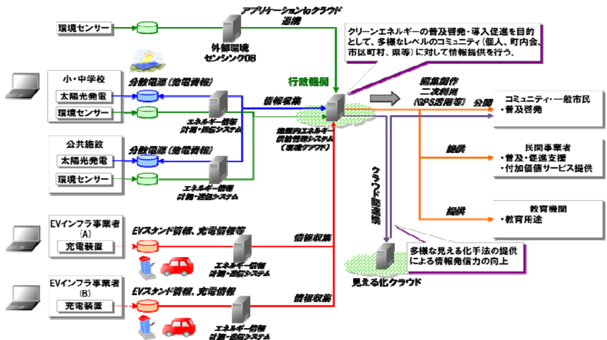
図 3-10 地域内エネルギー供給管理システムにおけるサービスモデル（例）
