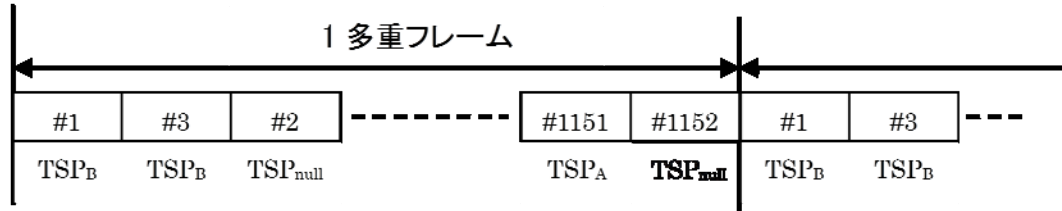
図 2.4-3 再多重されたトランスポートストリームの場合 (フルセグ型、モード 1、ガードインターバル 1/8 の場合)
