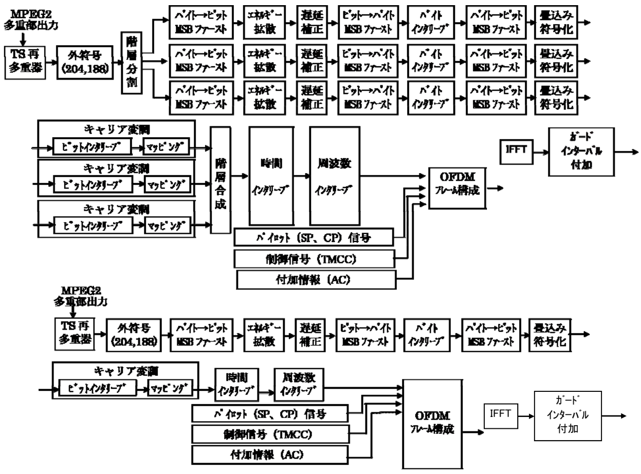
(b) ワンセグ型の伝送路符号化系統
