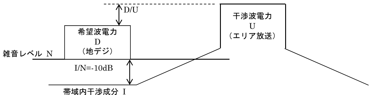
図3.2.3.1-2 混信保護基準に示すケースの希望波と妨害波の周波数とレベル関係の例
