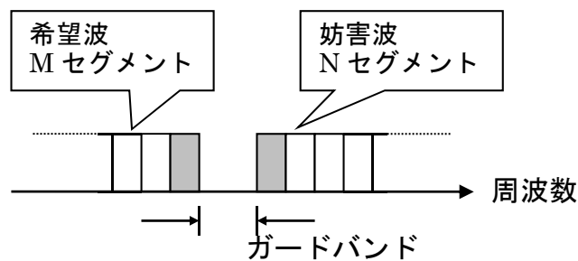
図3.2.3.2-1 希望波と妨害波の配置図
