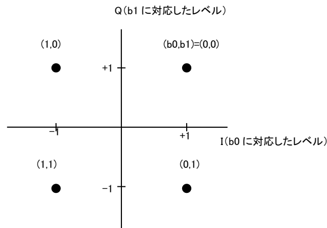
図 2.4-16 QPSK 位相図
