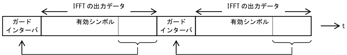
図 2.4-35 ガードインターバルの付加
