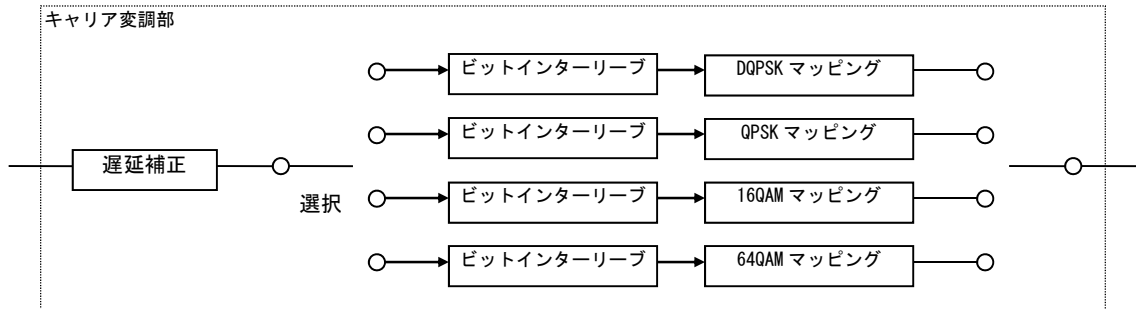
図 2.4-11 キャリア変調部の構成（フルセグ型）
