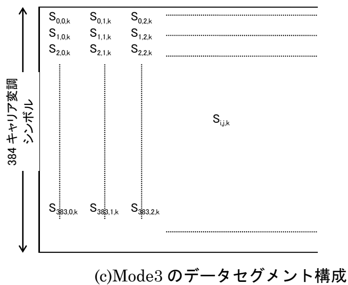
図 2.4-21 データセグメントの構成
