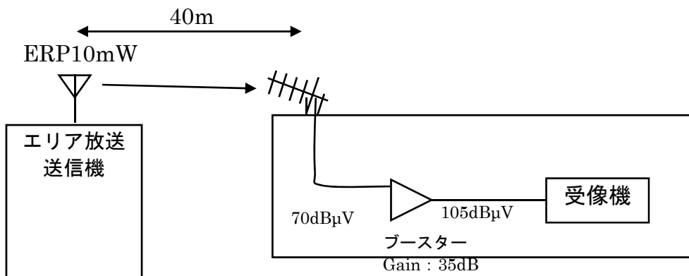
図3.3-1 エリア放送の受信モデル
