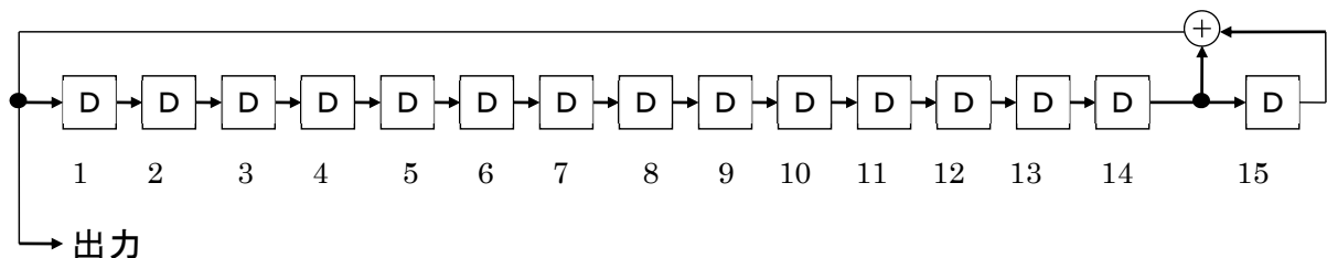
図 2.4-8 PRBS の生成回路
