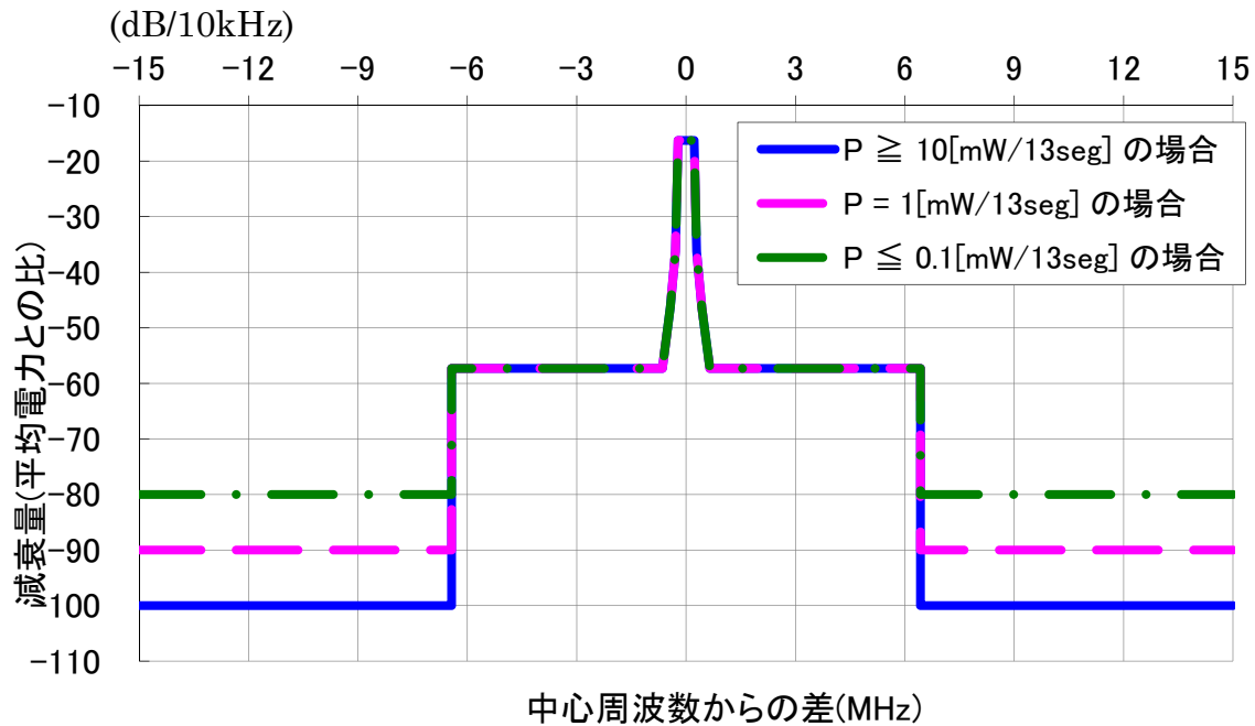
図表 2-10 ワンセグ型の送信スペクトルマスク
