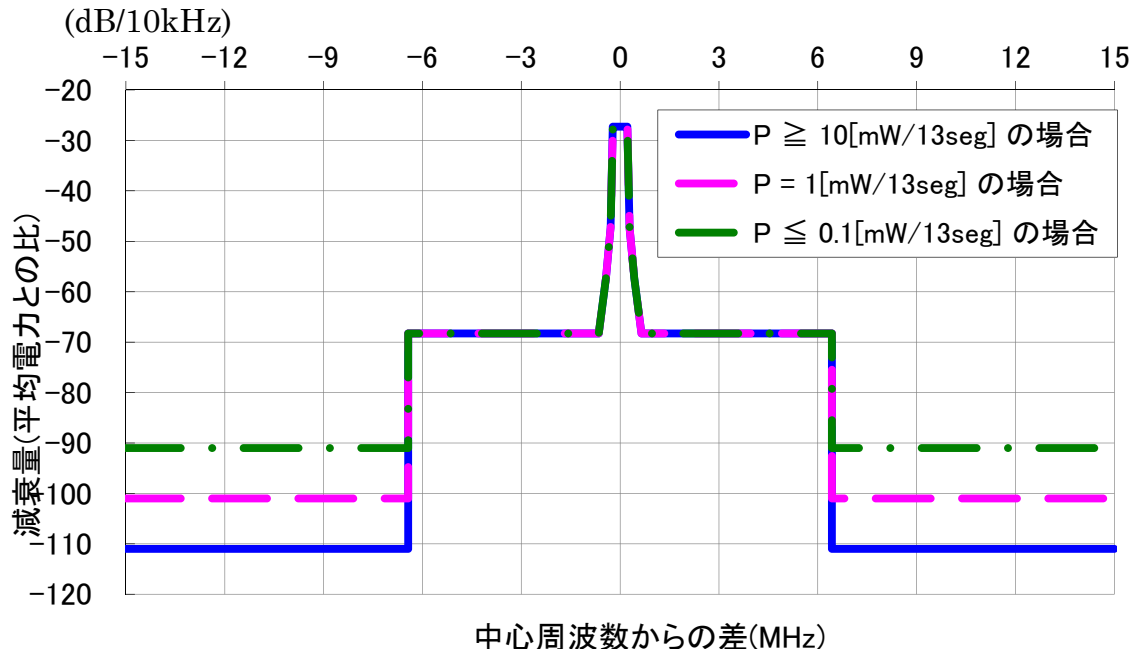
図表 2-12 バラセグ 13seg 送信を想定した場合を基準とした時の送信スペクトルマスク
