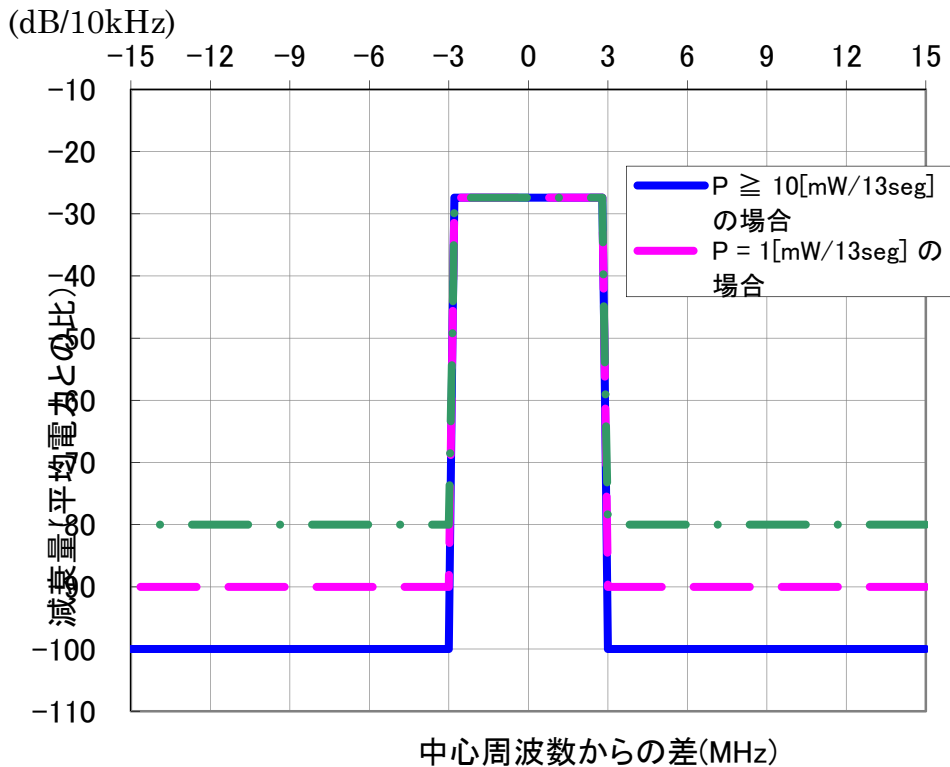
図表 2-8 隣接チャンネルを使用可能とするフルセグ型の送信スペクトルマスク
