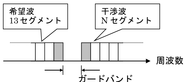
図3.2.3.1-1 希望波と妨害波の配置図
