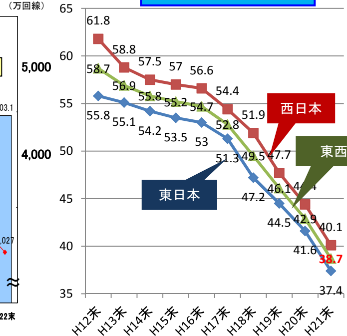
芯線使用率(メタル)の推移
