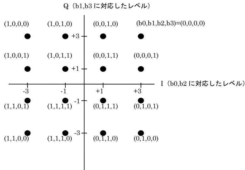
図 2.4-18 16QAM 位相図
