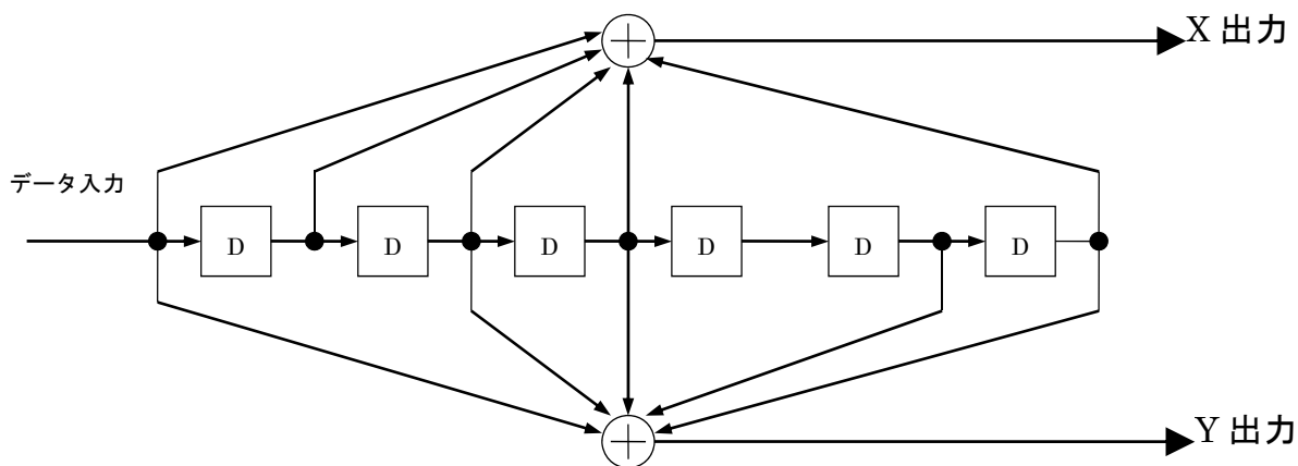
図 2.4-10 拘束長 k=7 、符号化率 1/2 の畳込み符号の符号化回路
