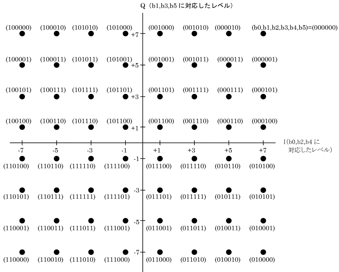
図 2.4-20 64QAM の位相図
