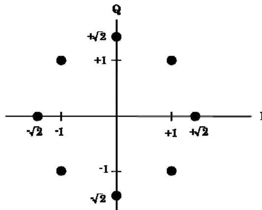
図 2.4-14 \pi/4 シフト DQPSK 位相図
