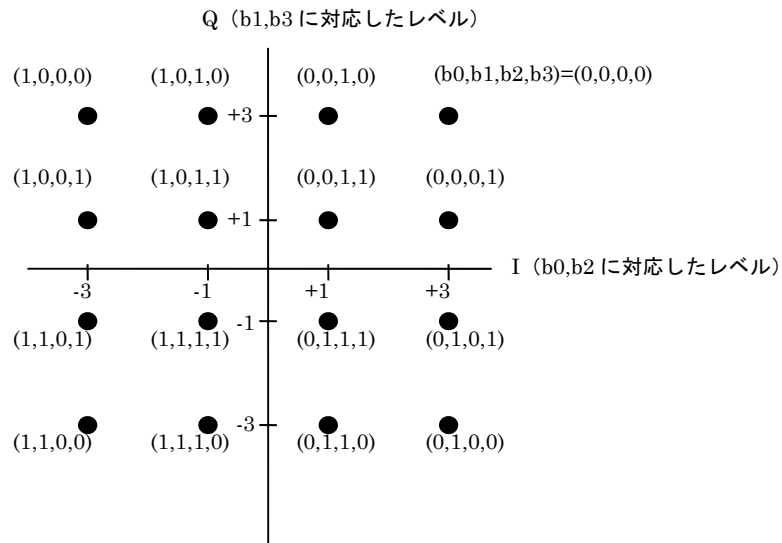
図 2.4-18 16QAM 位相図
