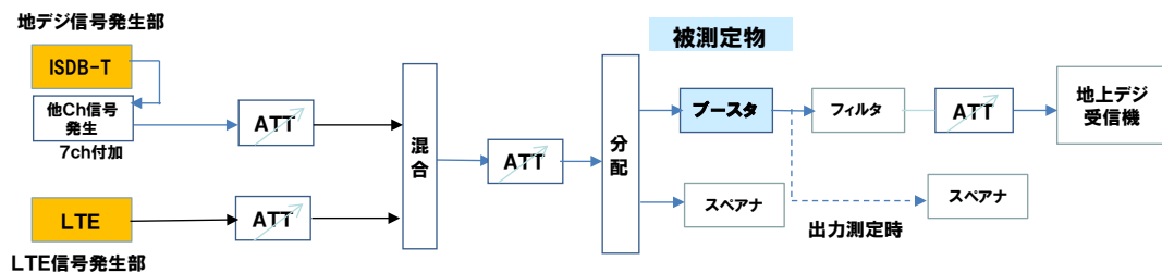
図. 添1-2-12 実験を行った評価測定系列
