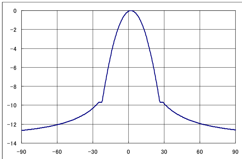
図. 添 1-10-1 DME 地上局のアンテナ特性 (垂直面)
