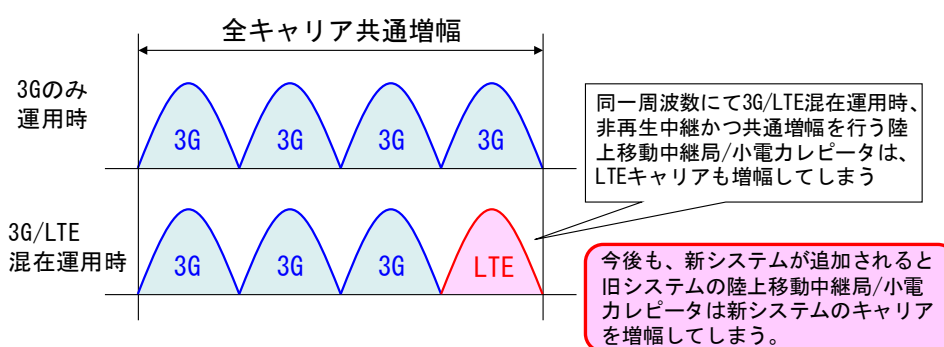
図4. 1-1 陸上移動中継局/小電力レピータにおける3G/LTE混在運用時のキャリア増幅
