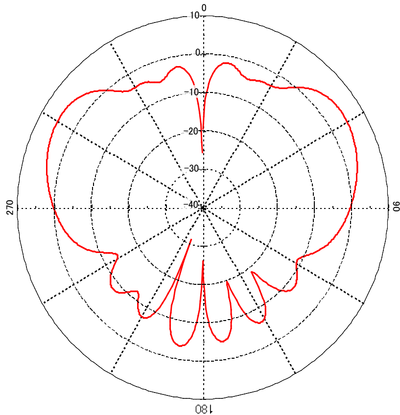
図 添1-3-5 ITS車載器アンテナパターン（モンテカルロシミュレーション）
