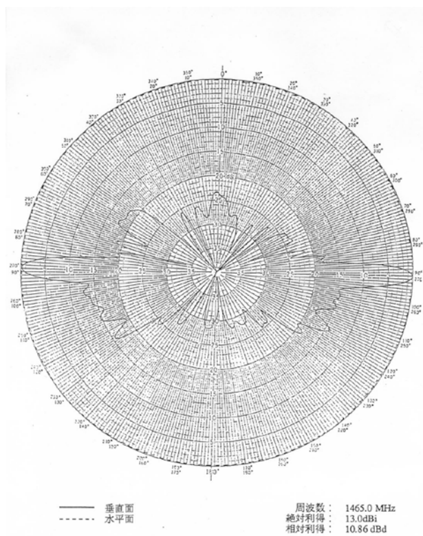
図. 添 1-7-6 MCAデジタル中継局の受信アンテナ特性 (実力値)
