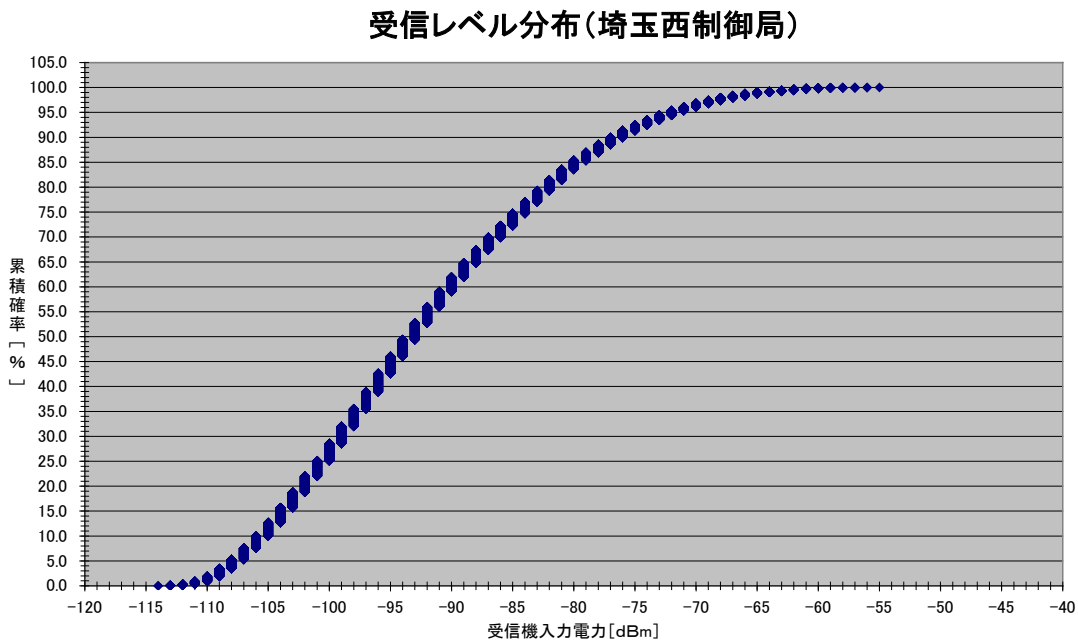
図. 添 1-7-8 MCAデジタル移動局の受信レベル分布データ
