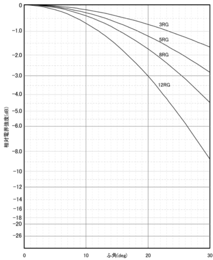
図. 添 1 - 2 - 8 極微小電力局受信ANT指向特性 (垂直) (12RGを使用)
