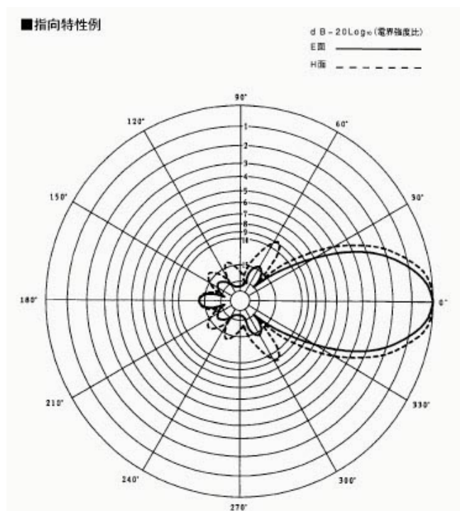
図. 添 1-7-7 MCAデジタル管理移動局の送受信アンテナ特性 (実力値)
