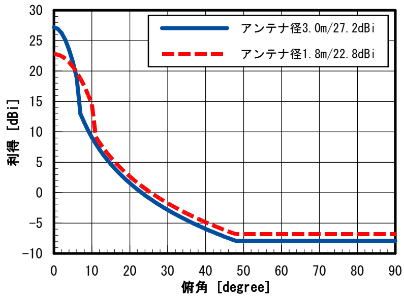
図. 添1-9-1 STLアンテナの指向特性
