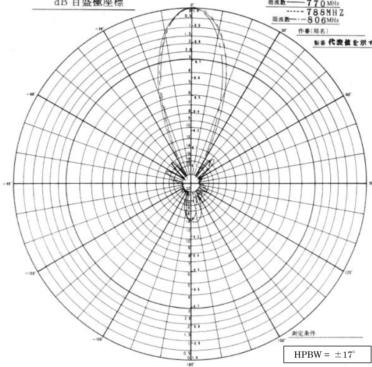
図. 添1-4-4 14素子八木単体放射パターン(E面)
