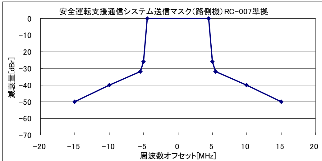
図 添 1-3-1 ITS路側機送信マスクパターン (モンテカルロシミュレーション)
