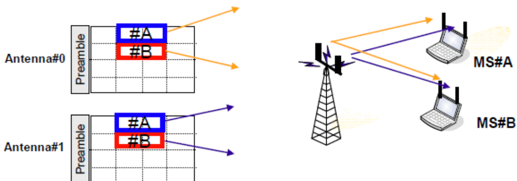
図1. 3. 3-2 バンドAMC+CL-MIMO
