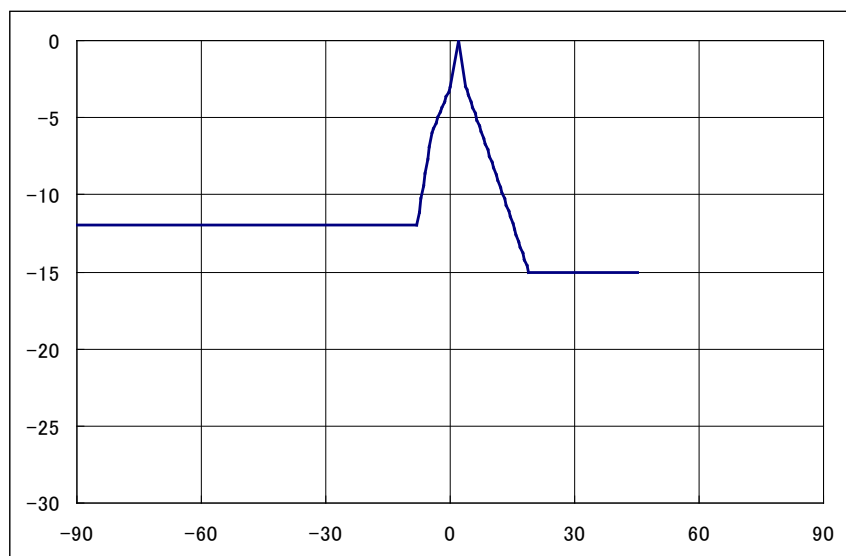
図. 添 1-10-3 SSR 地上局の受信アンテナ特性 (垂直面)
