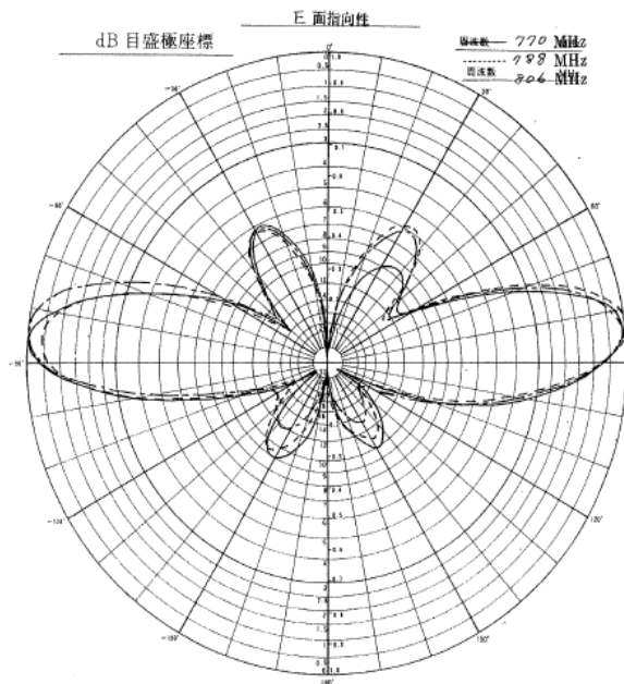
図. 添1-4-2 FPU受信アンテナ (無指向性)
