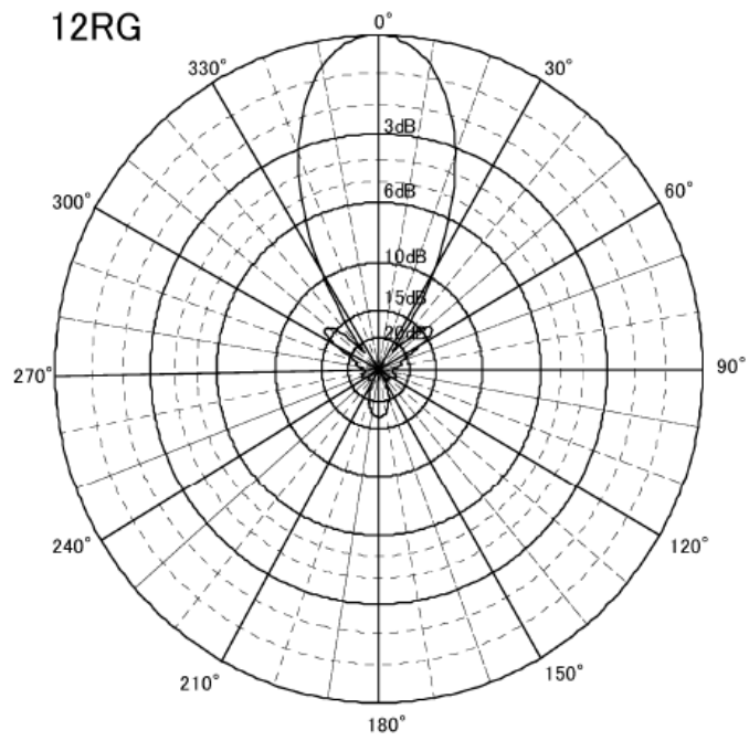
図. 添 1 - 2 - 7 極微小電力局受信ANT指向特性 (水平)
