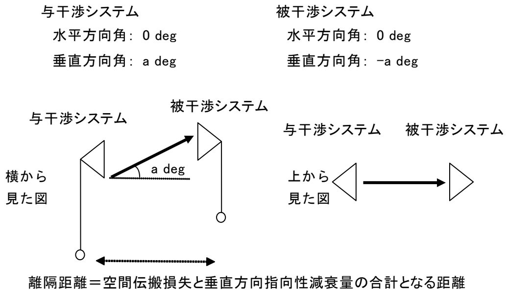
図 2. 1. 2-1 調査モデル
