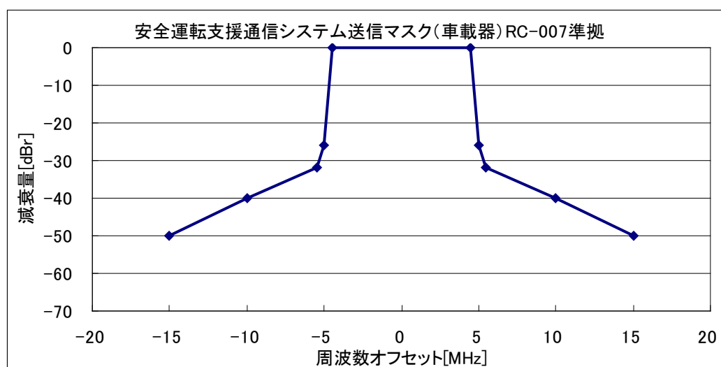
図 添 1-3-4 ITS車載器送信マスクパターン (モンテカルロシミュレーション)
