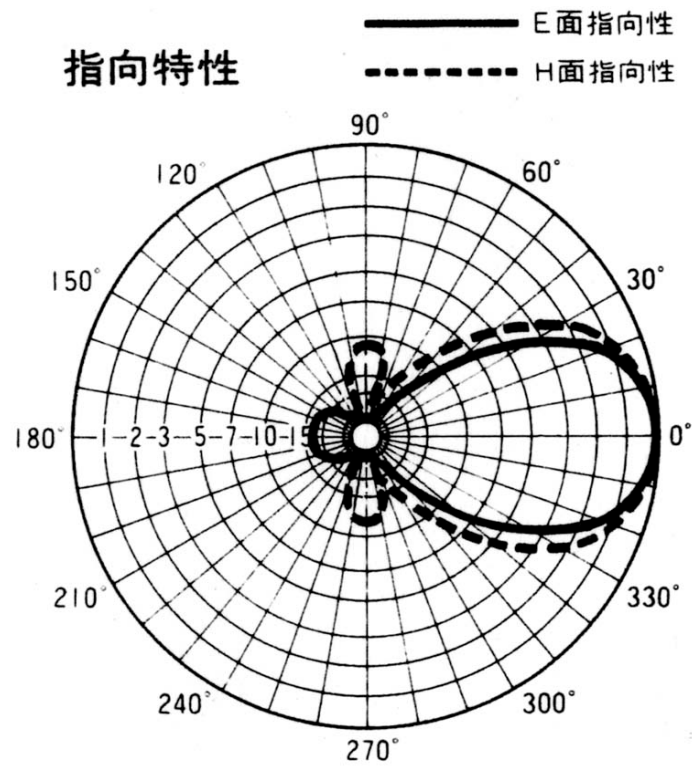
図. 添 1 - 7 - 4 MCA無線管理移動局の送受信アンテナ特性 (実力値)
