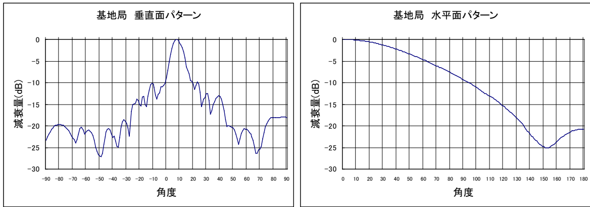
図. 添 1-12-1 PHS 基地局のアンテナ特性
