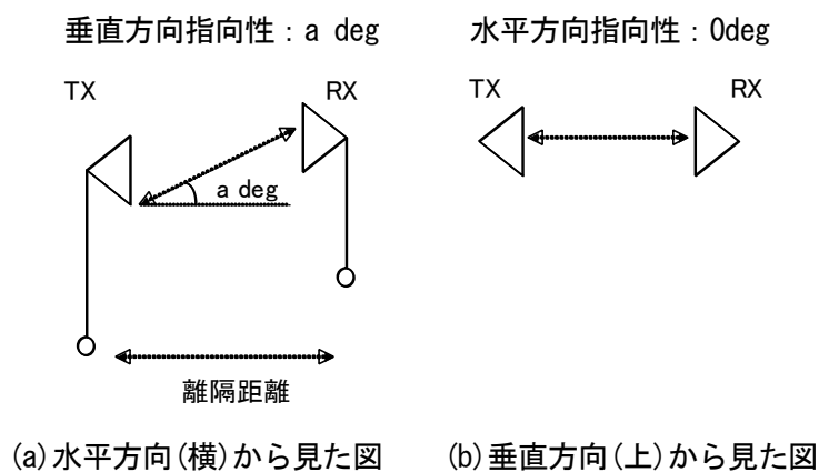
図 2. 5. 6-4 検討モデル2
