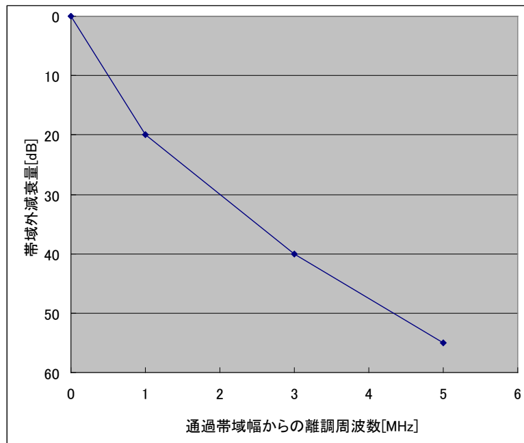
図. 添 1-7-5 MCAデジタル中継局受信フィルタ特性 (干渉形態を前提に調査した結果)
