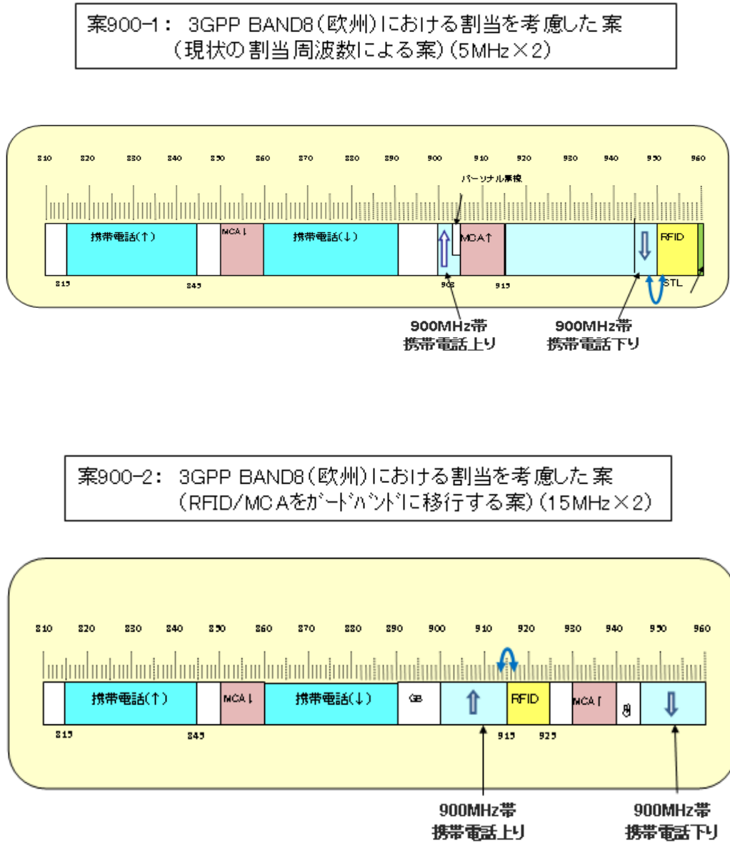
図 2. 5. 3-1 900MHz 帯周波数再編案
