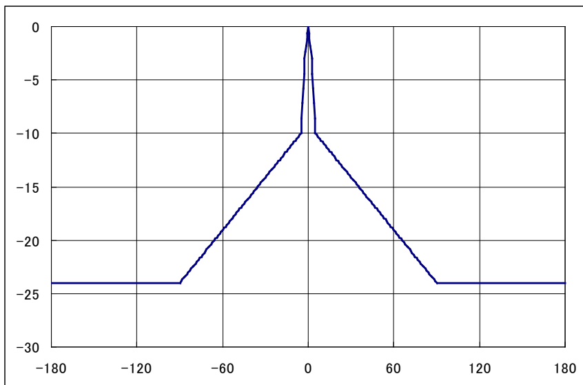
図. 添 1-10-2 SSR 地上局の受信アンテナ特性 (水平面)
