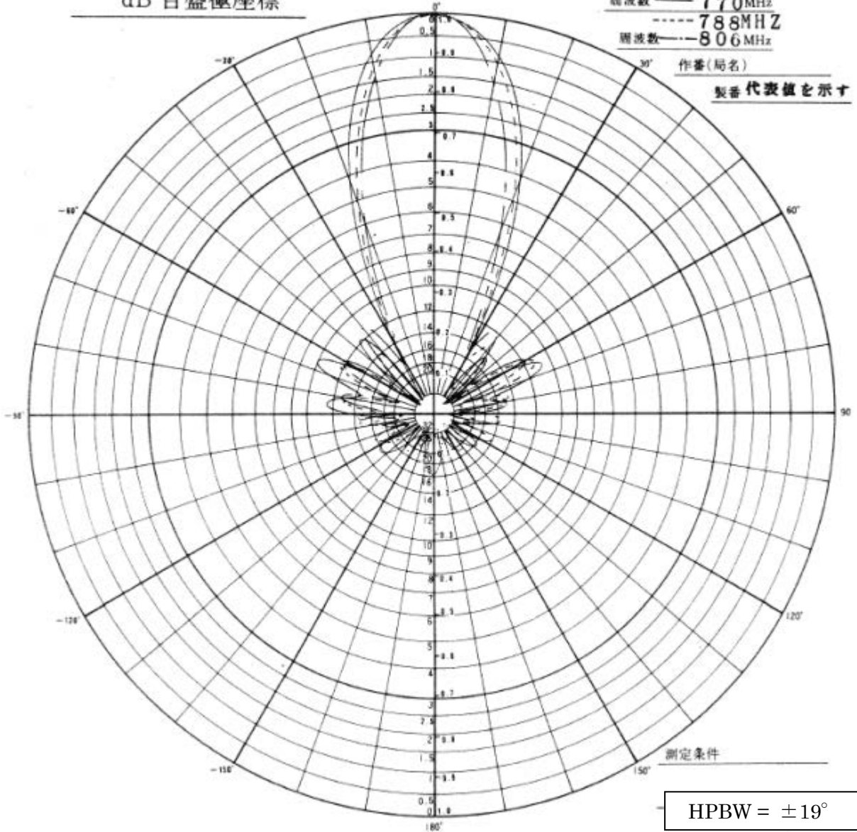
図. 添1-4-5 14素子八木単体放射パターン(H面)
