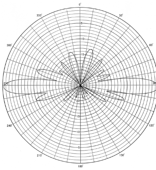
図. 添 1 - 7 - 1 MCA無線中継局の送受信アンテナ特性 1 (実力値)
