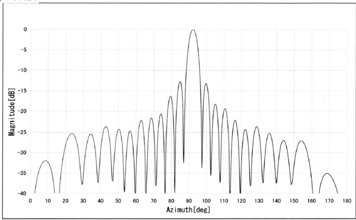
図. 添 1 - 7 - 2 MCA無線中継局の送受信アンテナ特性 2 (実力値)
