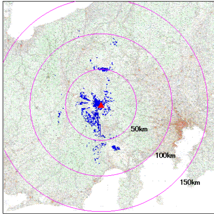
图 5. 4. 1. 1 - 1 野边山
