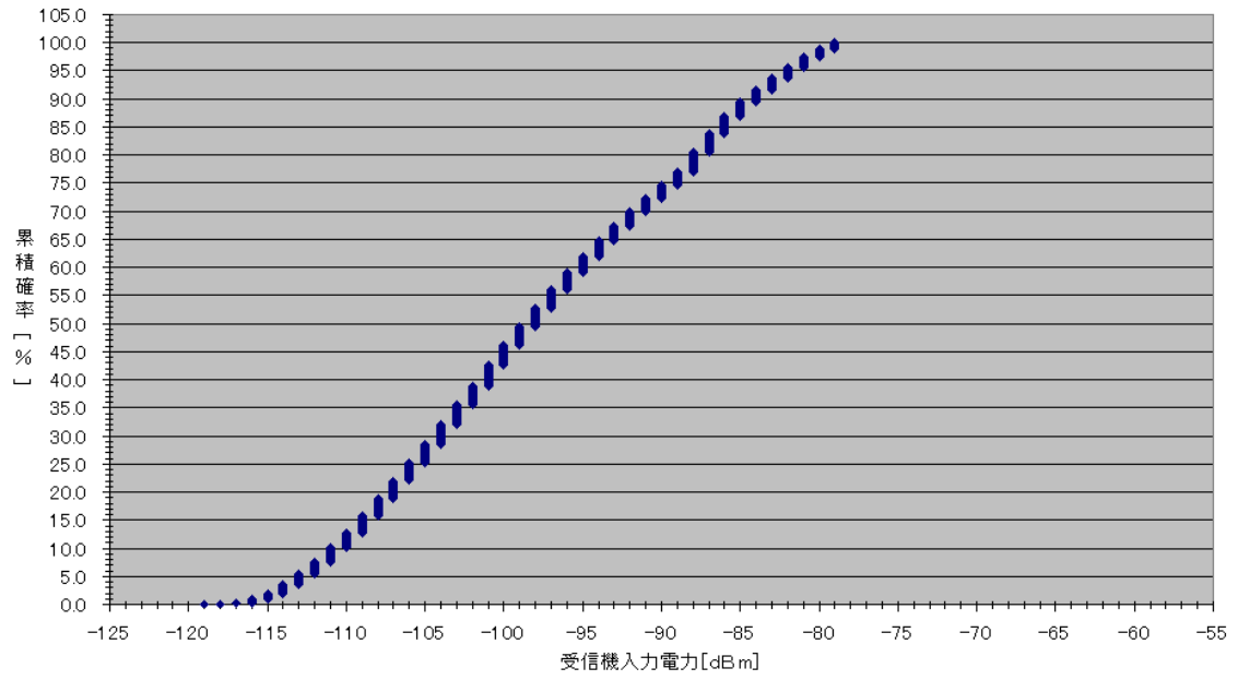
図. 添 1 - 7 - 9 MCAデジタル中継局の受信レベル分布データ
