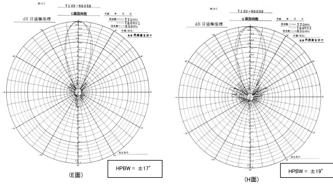
図. 添 1 - 4 - 3 FPU送信アンテナ
