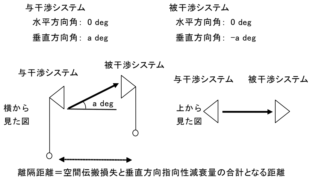
図5. 1. 2-1 調査モデル
