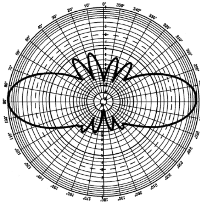
図. 添 1 - 7 - 3 MCA無線車載移動局の送受信アンテナ特性 (実力値)
