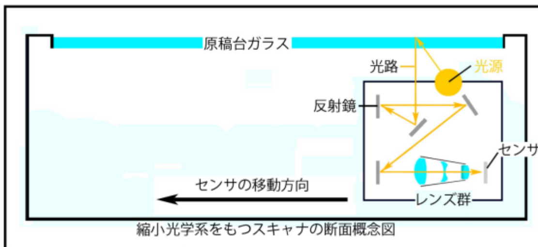
図 2 縮小光学系をもつスキャナの断面構造概念図
