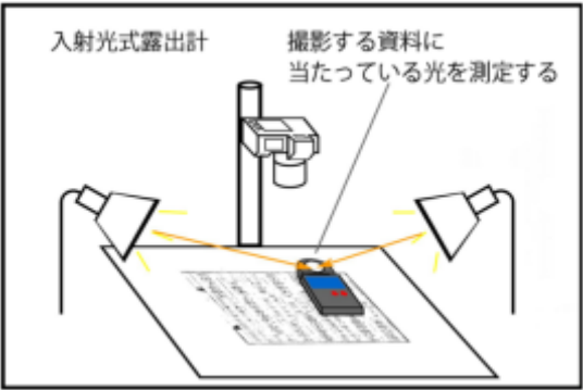
図 13 入射光式露出計を用いた露出の測定
