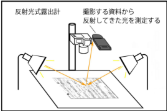
図 14 反射光式露出計を用いた露出の測定
