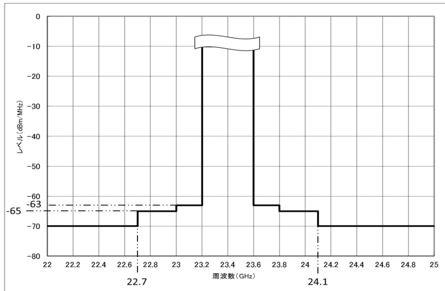
図 18 23GHz 帯無線伝送システム（汎用可搬型）の送信スペクトルマスク（絶対値）
