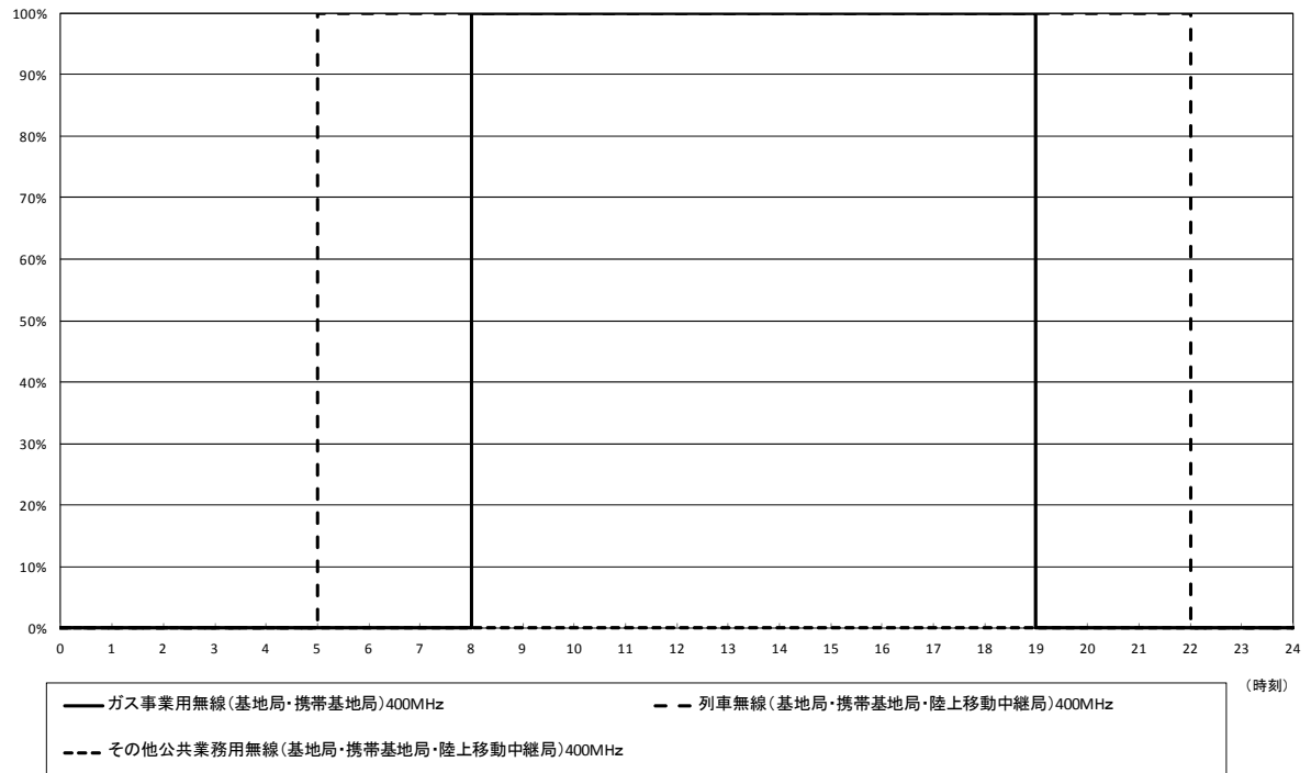
図表－９－６－４６ 運用時間帯の分布 (ガス事業用無線・列車無線・その他公共業務用無線 400MHz)【四国】
