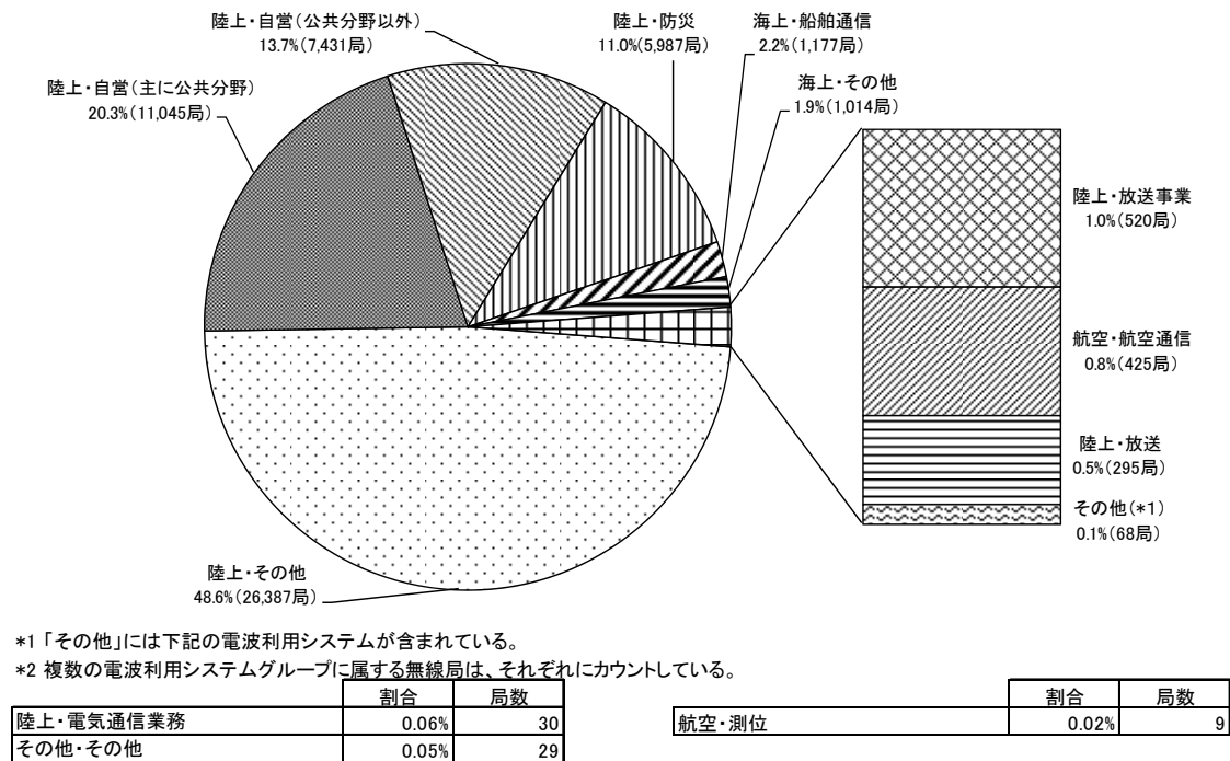
図表－９－４－６ 無線局数の割合及び局数【四国】
