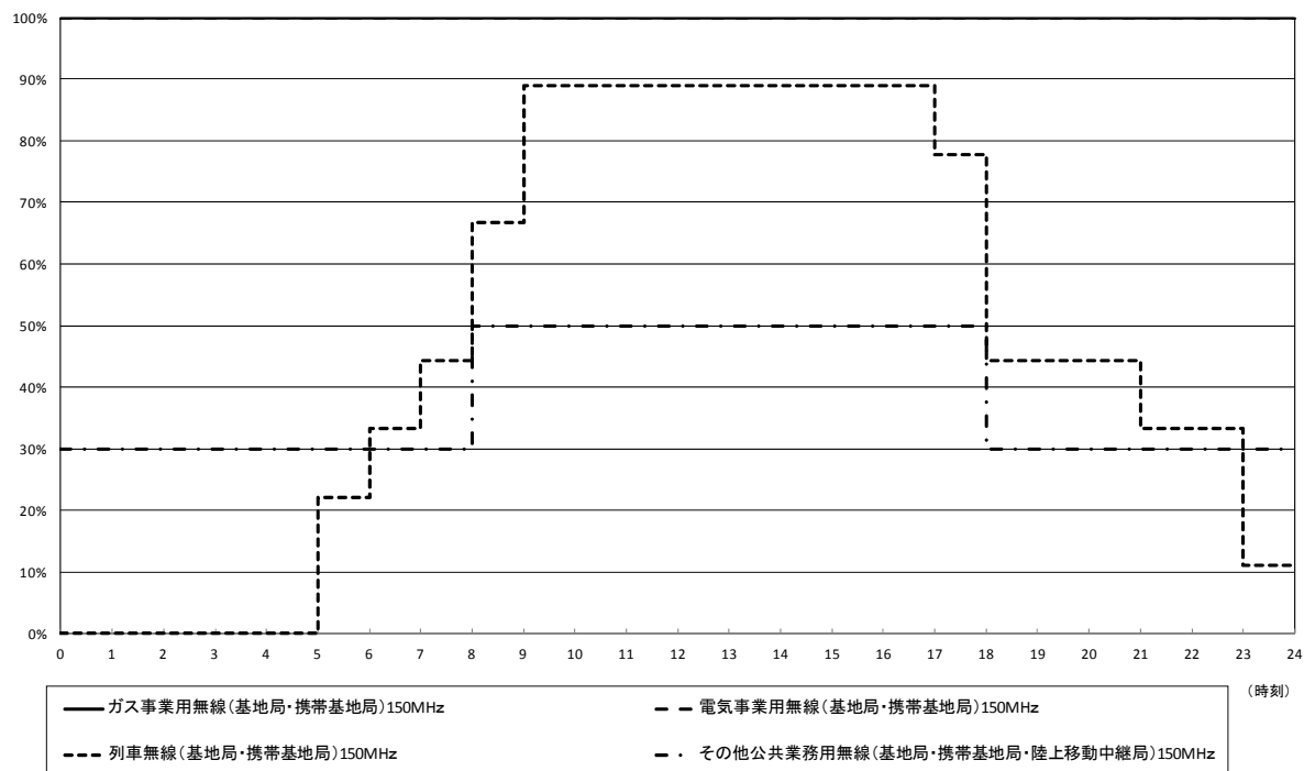
図表－９－４－１３ 運用時間帯の分布 (ガス事業用無線・電気事業用無線・列車無線・その他公共業務用無線 150MHz)【四国】
