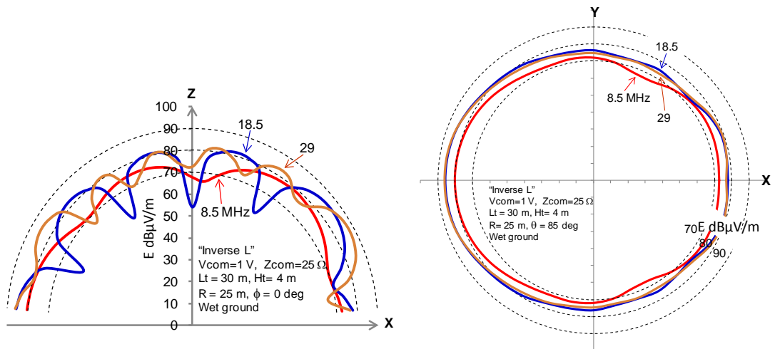
(a) 仰角方向指向特性
