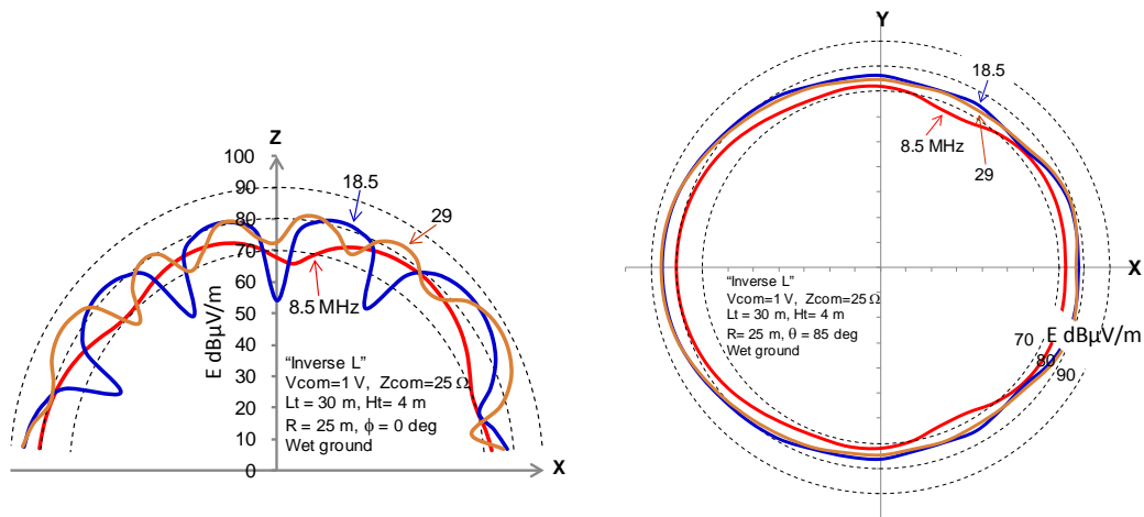
(a) 仰角方向の指向特性
