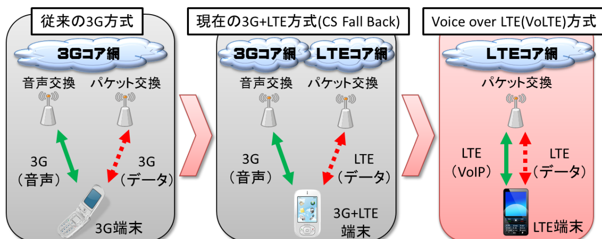
図1.1.1-3 IP移動電話へのネットワーク設備の移行イメージ(例:LTEの場合)
