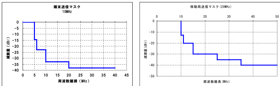
図. 参 1-1-4 移動局及び小電力レピータ送信マスク (10/20MHz システム)
