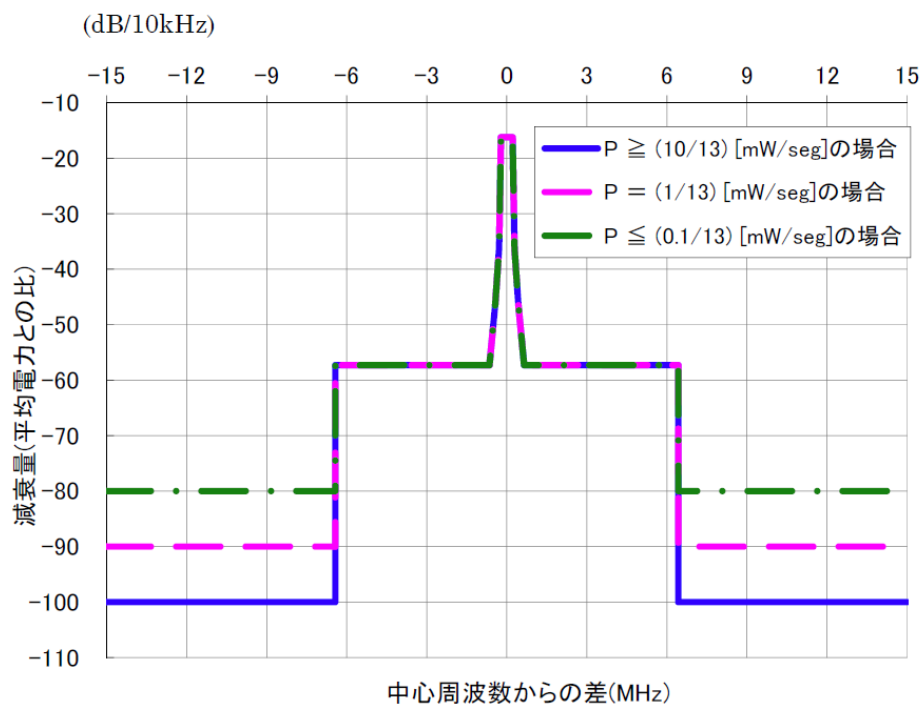
図5. 2. 1 ワンセグ型の送信スペクトルマスク
