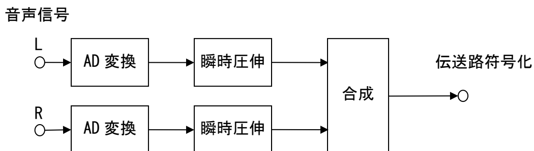
図 2-2 情報源符号化の基本構成（イヤ－・モニターの場合）
