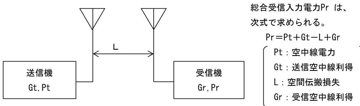
図1 標準伝搬路モデル
