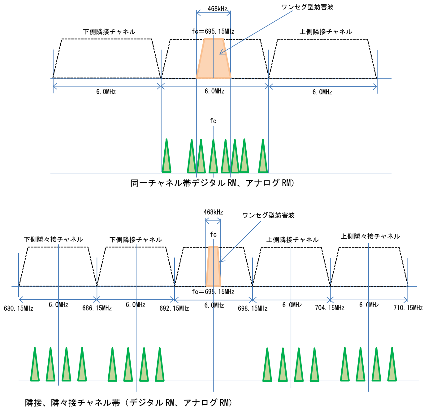
図 1 周波数配置
