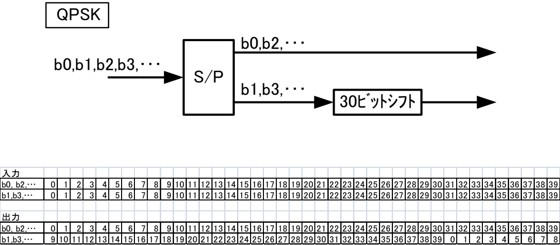
図 3-4 QPSK ビットローテーション
