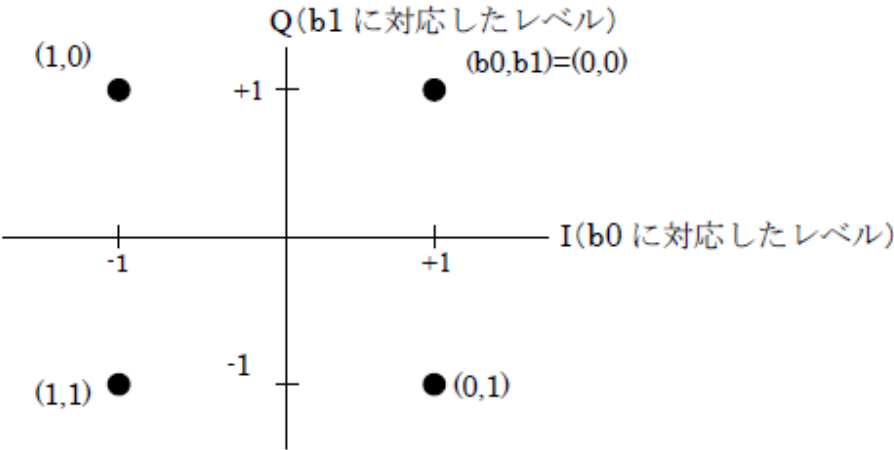
図 3-5 QPSK 位相
