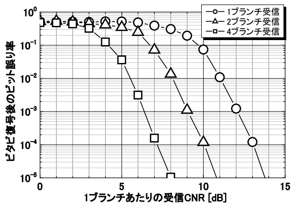
図4 標準マイク・イヤ－・モニター伝送モードのAWGN特性(16QAM)
