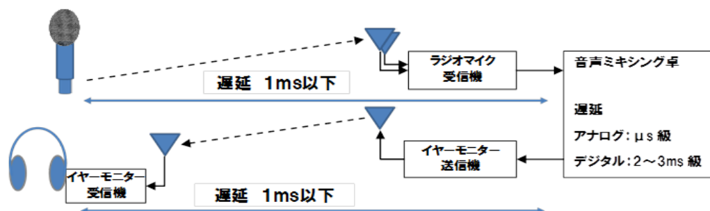
図3. 1. 3 特定ラジオマイク、イヤーク・モニター及びミキシング卓の遅延配分
