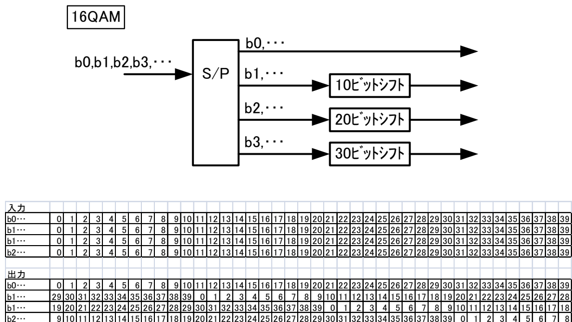
図 3-6 16QAM 変調系統図
