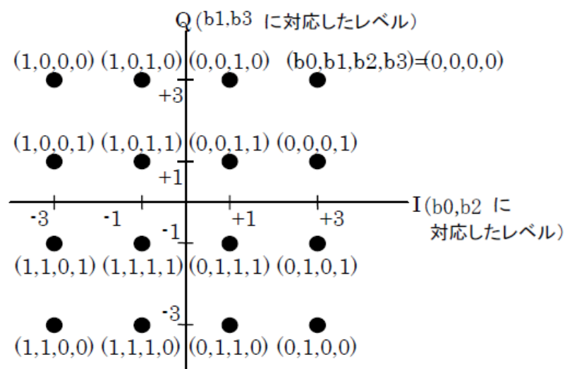
図 3-7 16QAM 位相図
