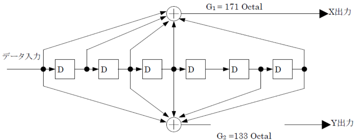
図 3-2 拘束長 k=7、符号化率 1/2 の原符号の符号化回路
