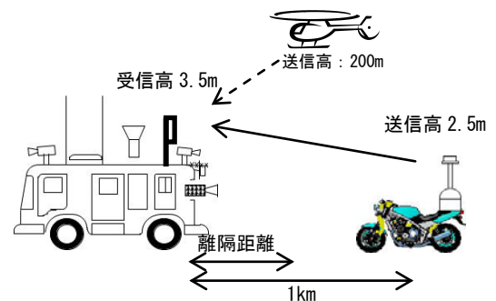
図 16-1 特定小電力無線局に対する FPU 被干渉モデル
