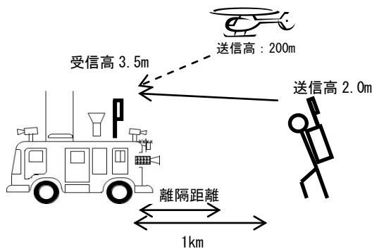
図 16-1 特定小電力無線局に対する FPU 被干渉モデル
