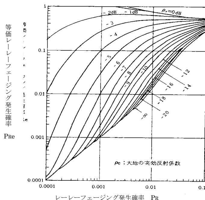
反射波がある場合の等価レーレーフェージング発生
