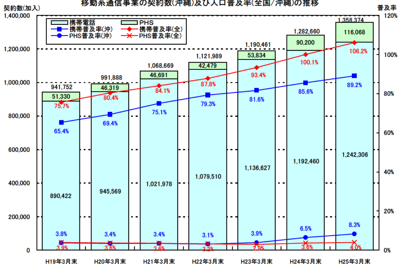
移動系通信事業の契約数(沖縄)及び人口普及率(全国/沖縄)の推移
