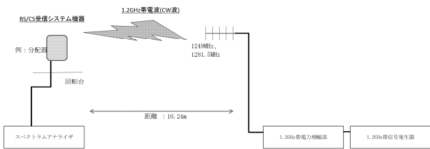
図1 電波暗室における測定系統
