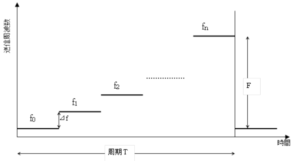
図 2.3-5 周波数コード変調送信波形の一例
