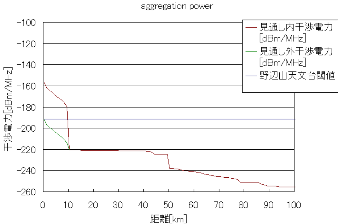
図6-1 干渉電力距離特性（普及率0.3%）
