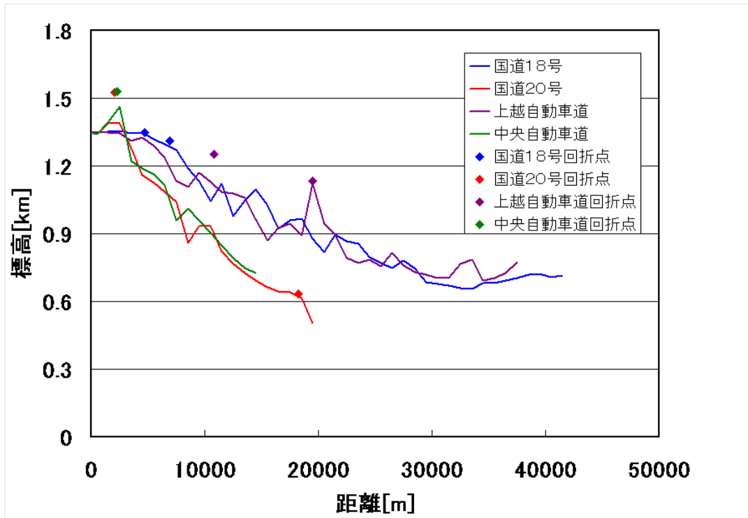
図 7-2 主要道路までの地形断面図 (1km 刻み)。点は回折損計算に使用したエッジを示す。
