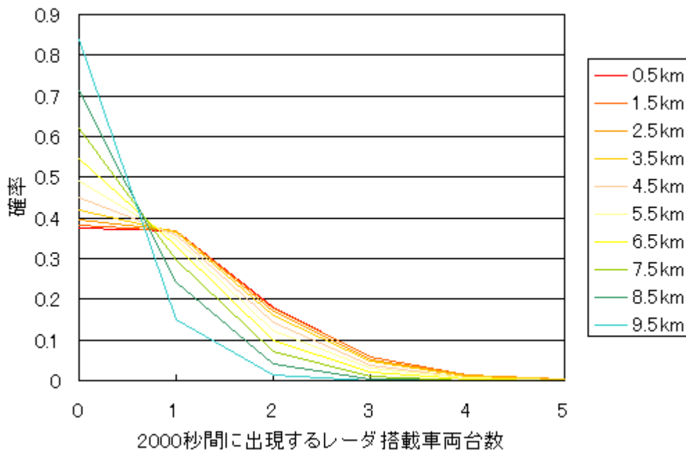
図 8-3 交通量パラメータを基にした半径 10.5km から各離隔距離まで 2000 秒間中出现するレーダ搭載車両台数の確率分布。
