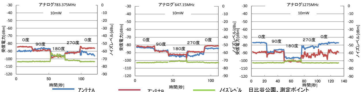
図2 屋外伝搬特性（800MHz帯、FM帯、1.2GHz帯の比較）の比較（測定場所：日比谷公園）
