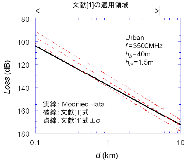
図 参2. 1. 3-1 距離特性の比較結果 (市街地)
