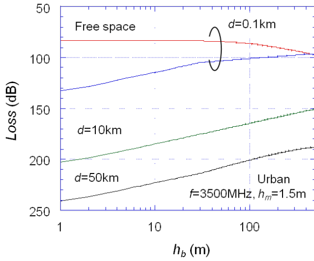
图 参 2. 1. 2-3 基地局高特性
