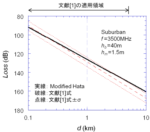
図 参2. 1. 3-3 距離特性の比較結果 (郊外地)
