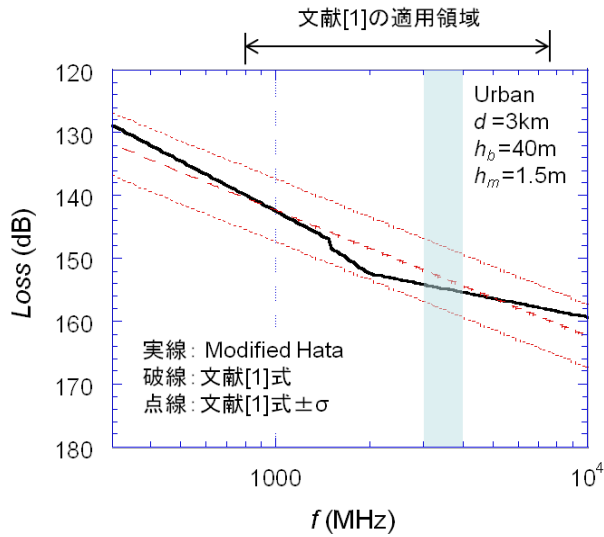
図 参2. 1. 3-2 周波数特性の比較結果 (市街地)
