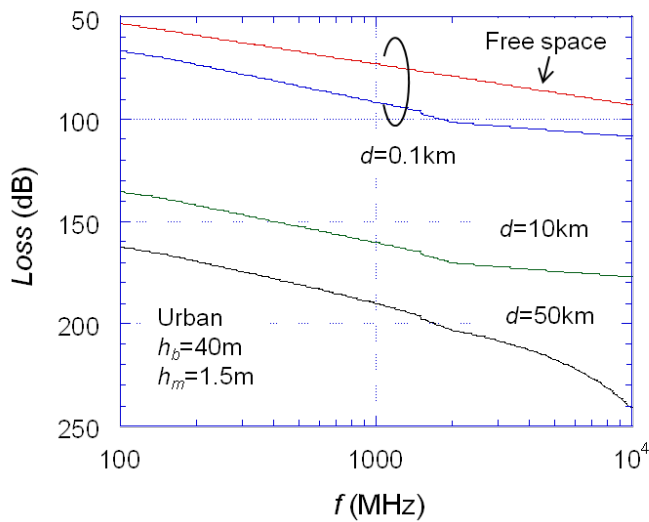
図 参2. 1. 2-2 周波数特性
