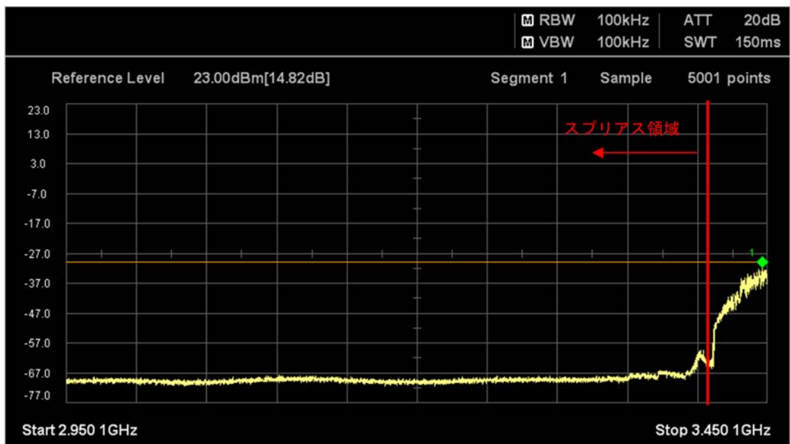
図 参 7. 4. 2-20 送信機のスプリアス特性 (CA f=3. 47GHz 送信時下側 MPR=0dB)
