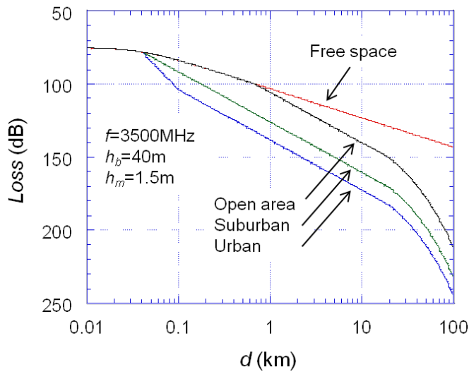
図 参2. 1. 2-1 距離特性
