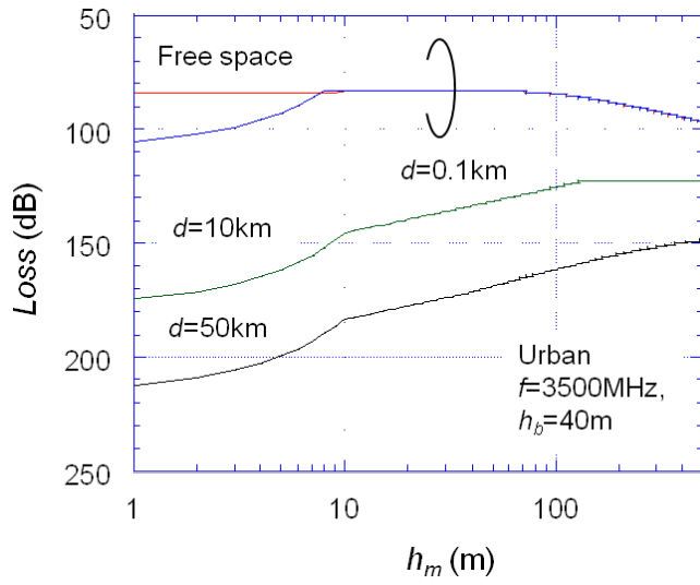
图 参 2. 1. 2-4 陸上移動局高特性
