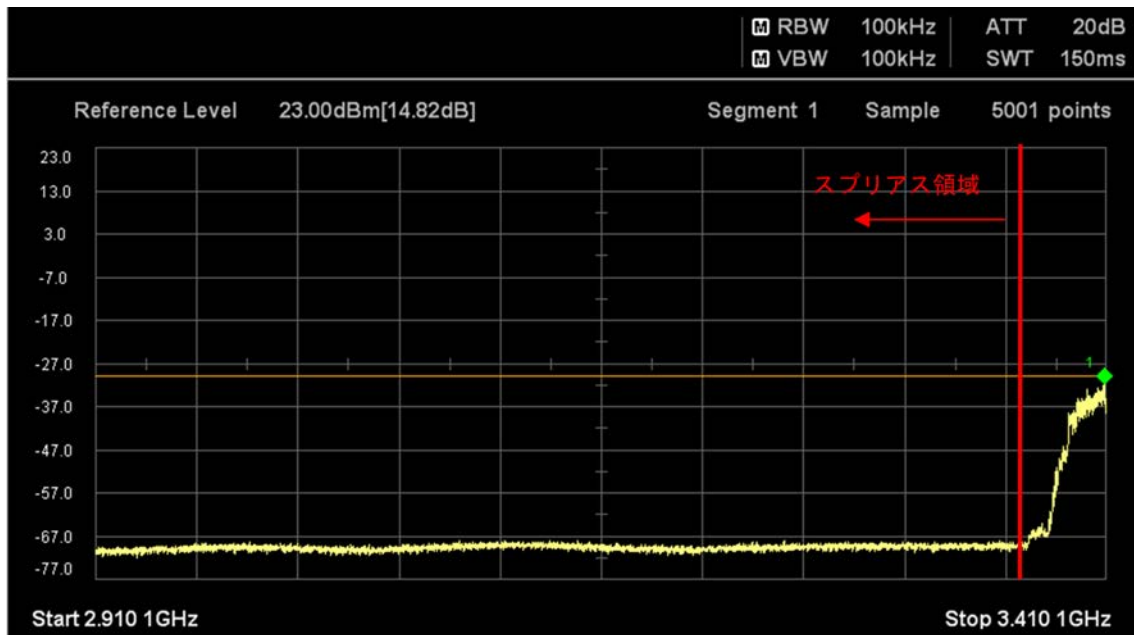
図 参 7. 4. 2-18 送信機のスプリアス特性 (CA f=3. 43GHz 送信時下側 MPR=0dB)
