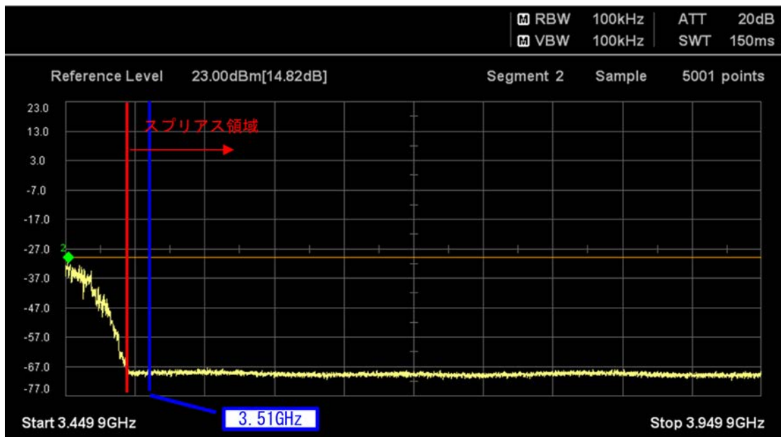
図 参 7. 4. 2-19 送信機のスプリアス特性 (CA f=3. 43GHz 送信時上側 MPR=0dB)
