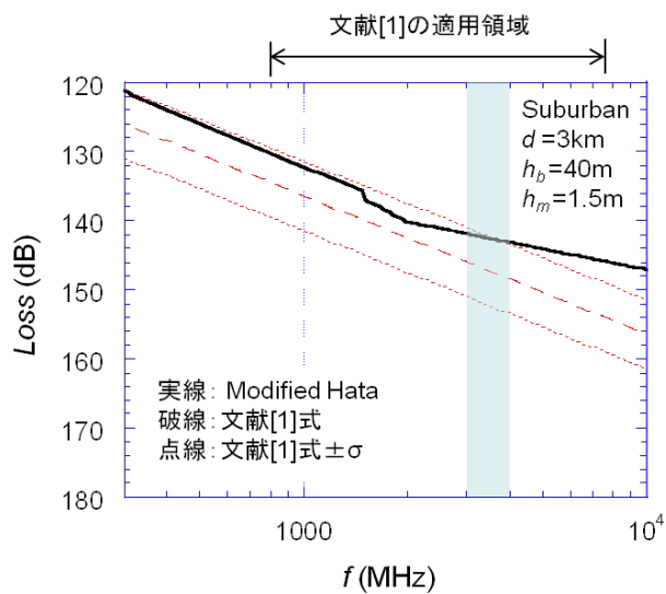
図 参2. 1. 3-4 周波数特性の比較結果 (郊外地)
