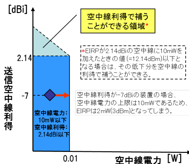
図 3 - 2 空中線利得と空中線電力の関係
