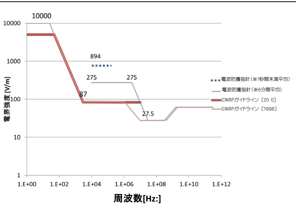
【電界強度】
