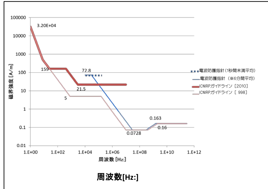
【磁界強度】
