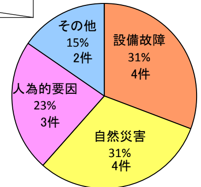
平成24年度放送停止事故の発生原因別件数
