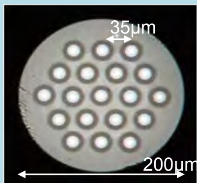
19コアファイバ
