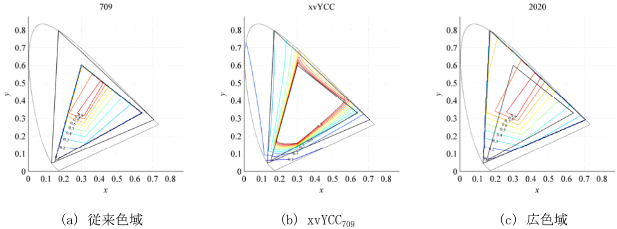
図 1 表色系と色域
