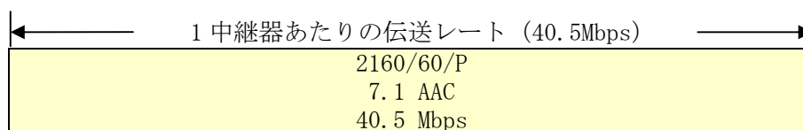
図 3.2-3 4K（60P）とロスレス音声システムの帯域利用イメージ
