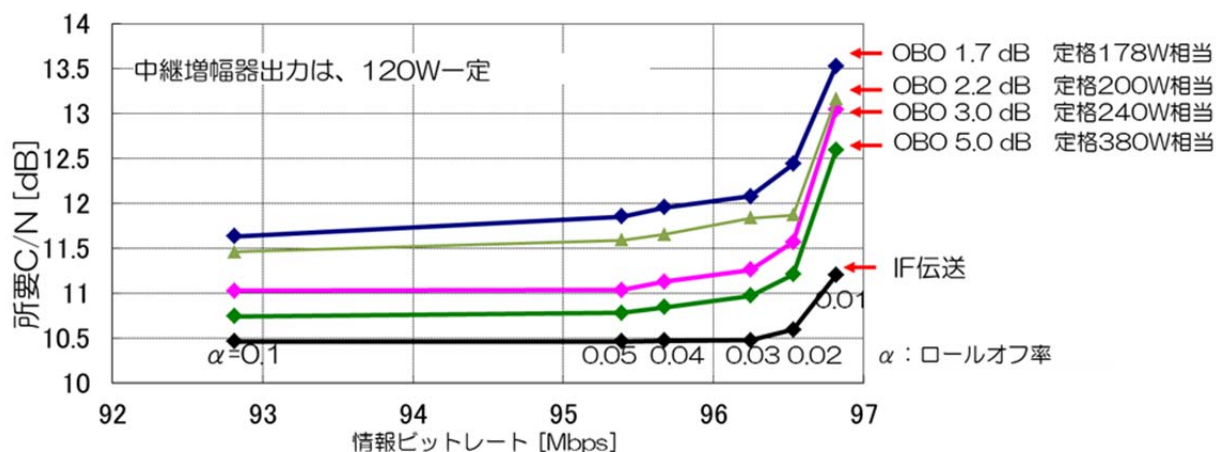
図 2. 2. 1-18 ロールオフ率及び中継器動作点に対する 16PSK の性能
