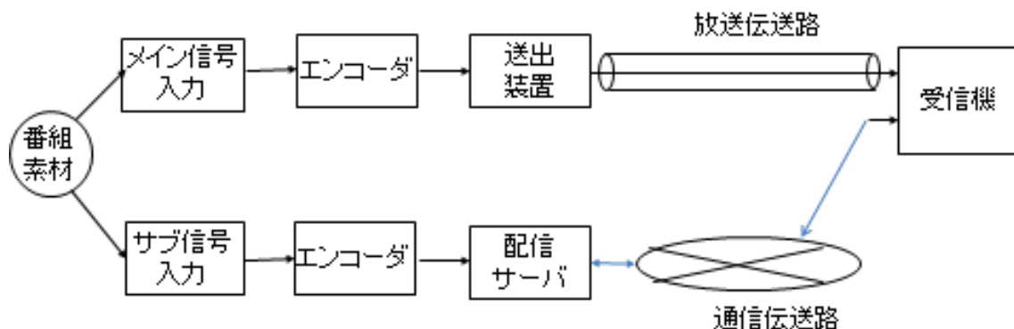
図1 放送・通信ハイブリッド伝送のシステム構成
