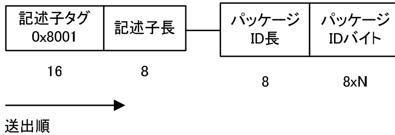
図 2.3-20 イベントパッケージ記述子の構成
