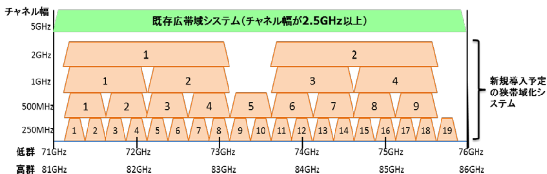
図 2-2 狭帯域システム制度化初期のチャネル配置案
