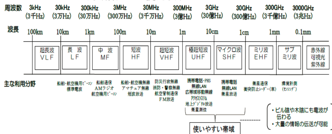
周波数ごとの使用状況
