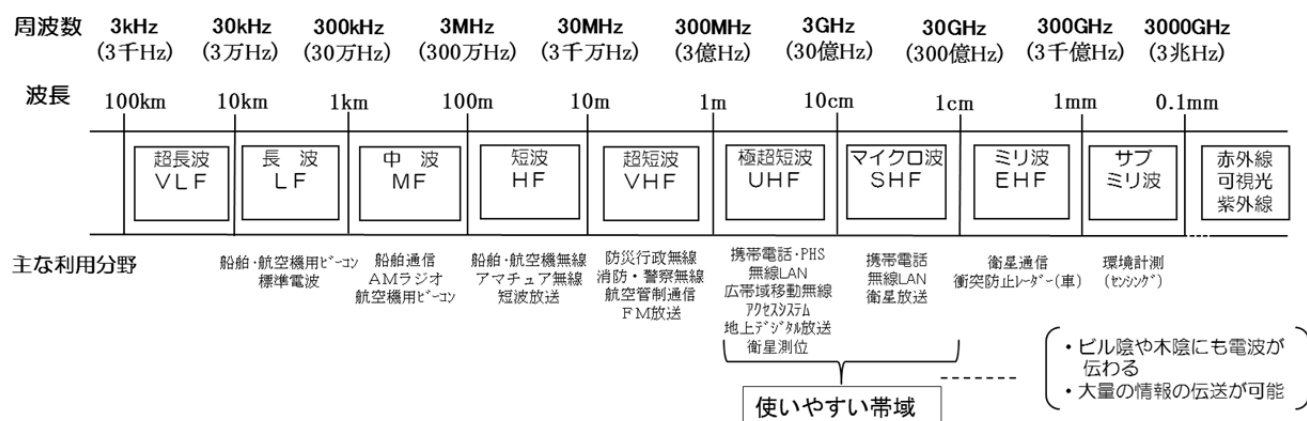
図表1-1-1 周波数利用状況
