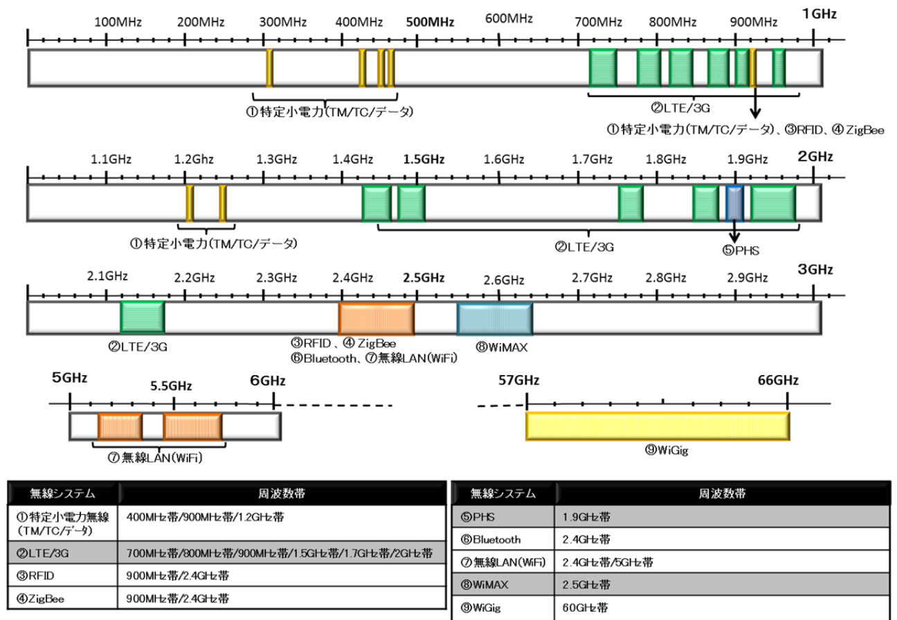
図表 2－1－3 M2M, IoT に利用可能な周波数
