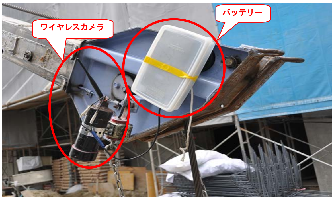
【クレーン車先端部に取り付けられたワイヤレスカメラ】
