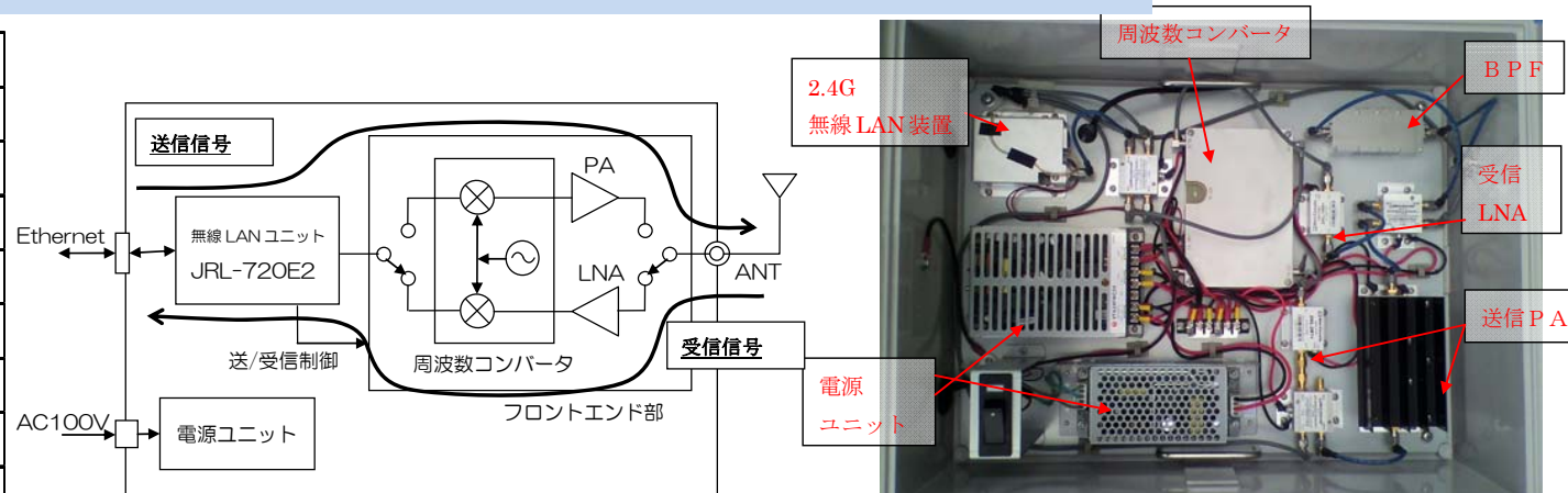
試作装置のブロック図
