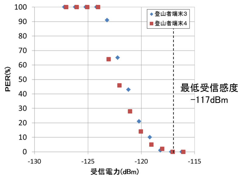
受信電力－PER特性
