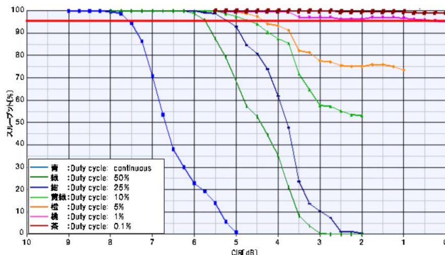
図 付 7-2 アクティブタグシステム与干渉 Duty 比に対する所要 CIR
