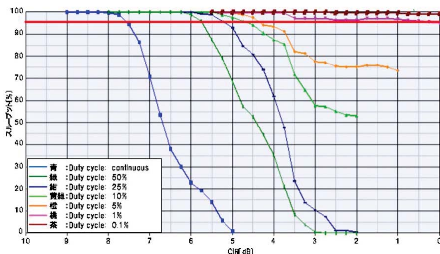
図 6-10 アクティブタグシステム与干渉デューティ比に対する所要 CIR
