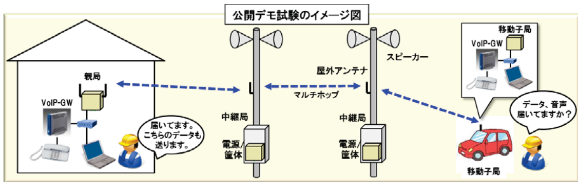
図 付 7- 1 公開デモ試験の構成
