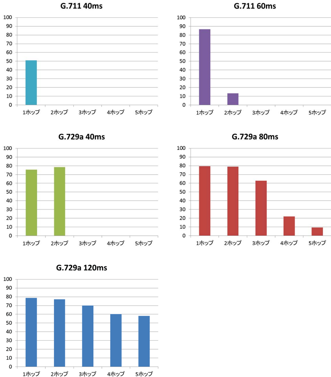
図 4-4 同時通話 1 回線の場合の各コーデックの R 値
