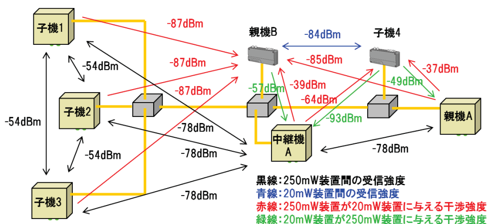
図 6-5 各無線局間の受信強度
