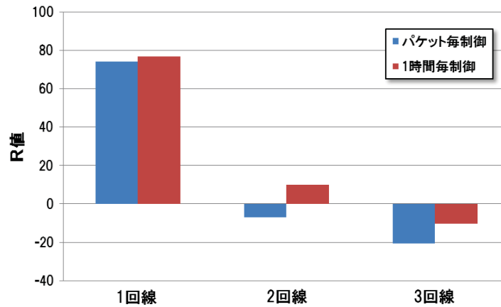
図 4-10 2 ホップ時におけるデューティ制御方式の比較
