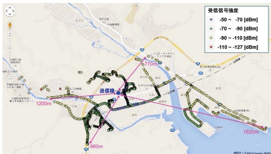
図 付 3- 4 920MHz 帯無線装置の受信信号強度
