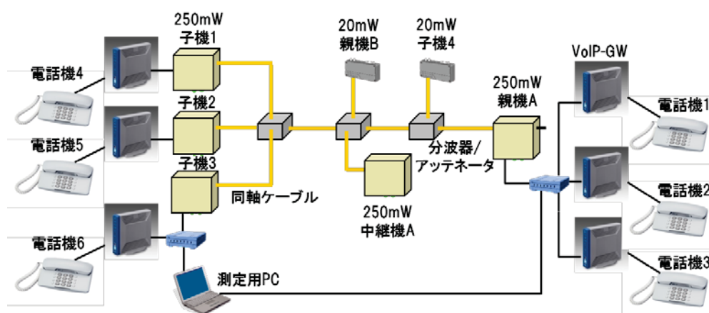
図 6-4 ラボ内試験環境の構成
