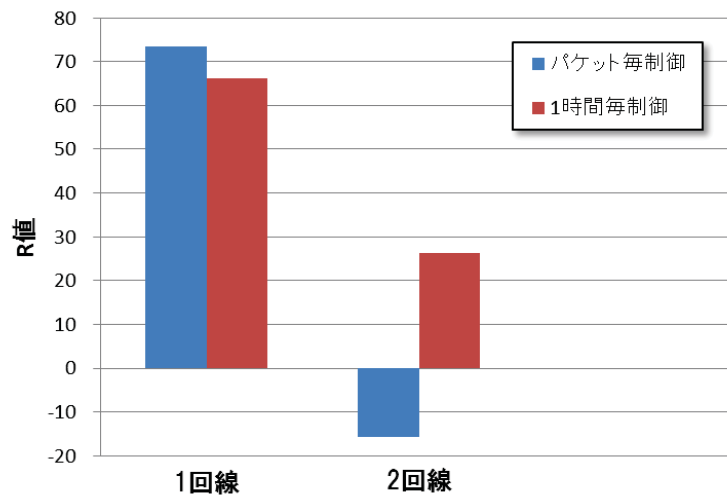
図 5-12 2 ホップの測定結果(10 分間)
