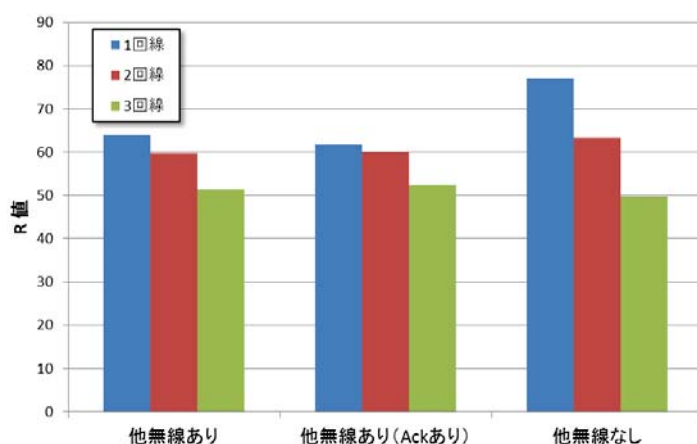
図 6-8 20mW 無線局からの被干渉 (R 値)
