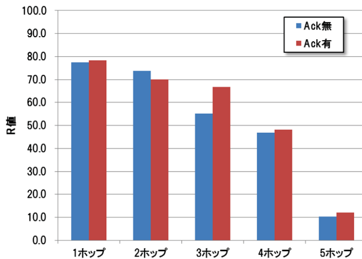
図 5-6 1 回線時におけるホップ数の評価
