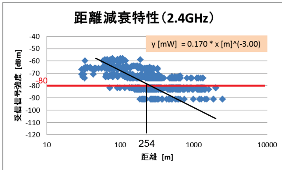
図 付 3- 7 2.4GHz 帯無線装置の許容受信入力レベルと通達距離
