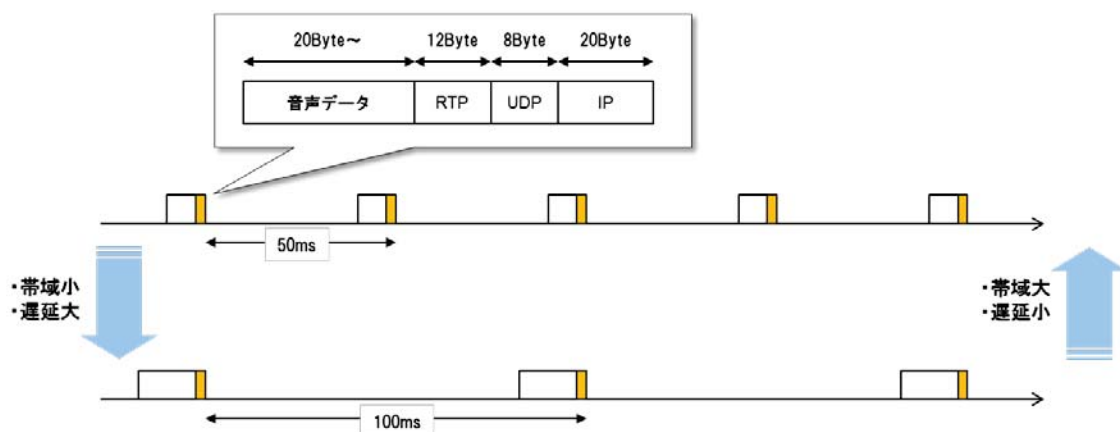
図 3-1 送信間隔と使用帯域、遅延の関係
