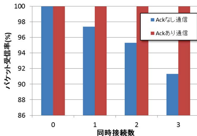
図 6-6 20mW 無線局への与干渉
