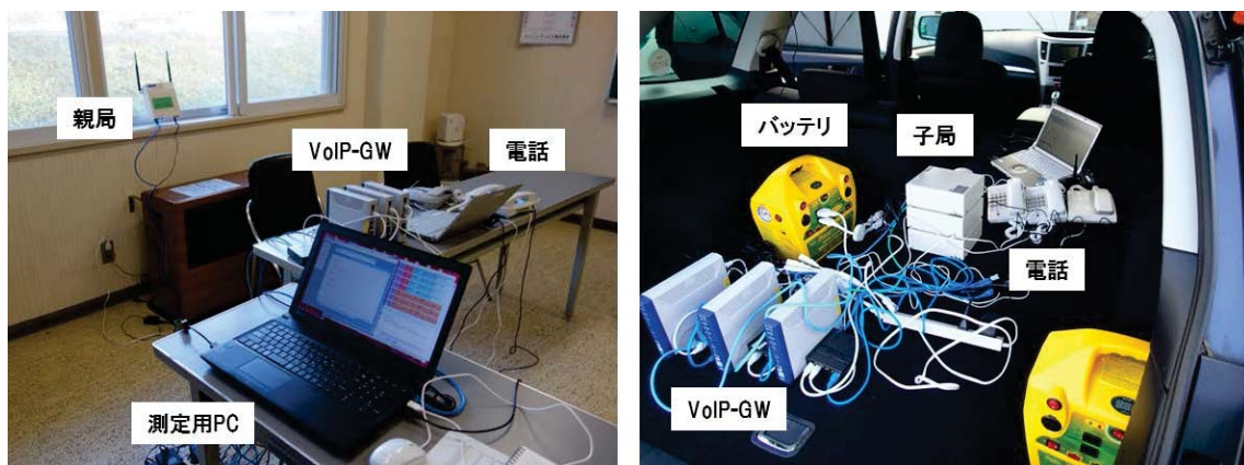
図 5-2 屋内親局(左図)と移動子局(右図)設置の様子
