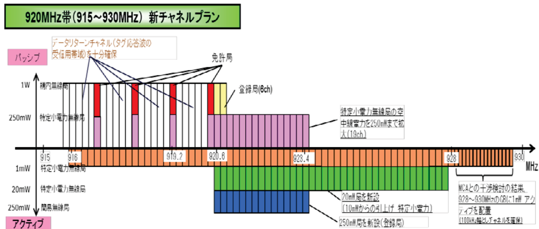
図 2-6 920MHz 帯における新チャンネルプラン
