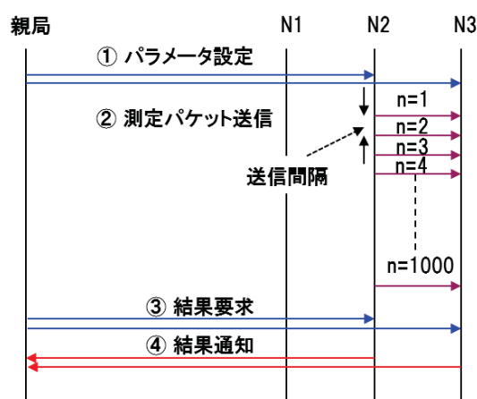
図 5-4 電波伝搬の測定手順
