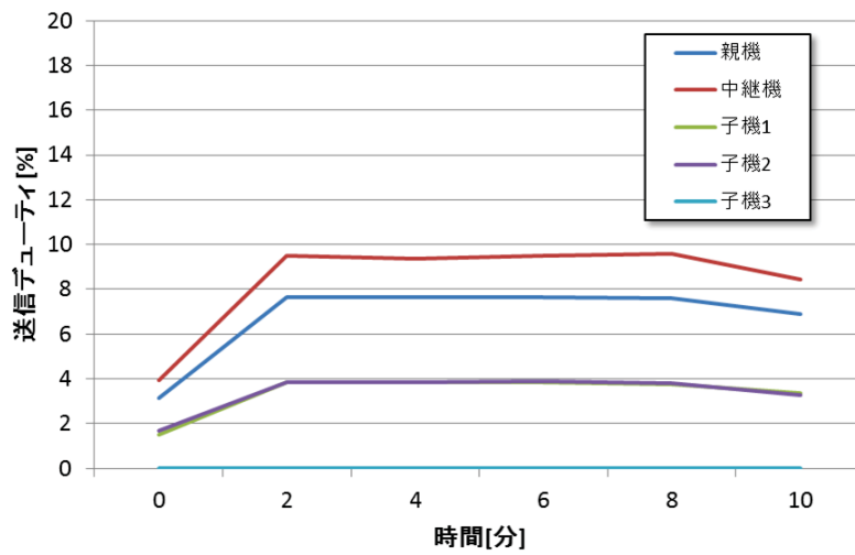
図 4-12 パケット毎制御方式のデューティの時間変化
