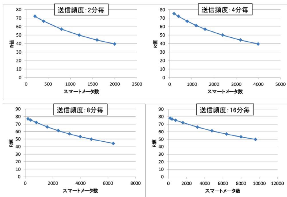
図 6-9 スマートメーターの設置密度に対する R 値
