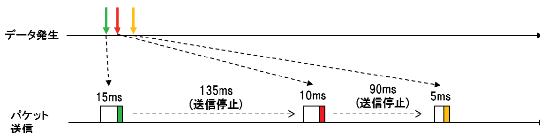
図 3-3 パケット毎に行うデューティ制御
