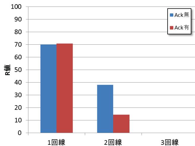
図 4-9 3 ホップ時における複数通話回線の R 値の比較
