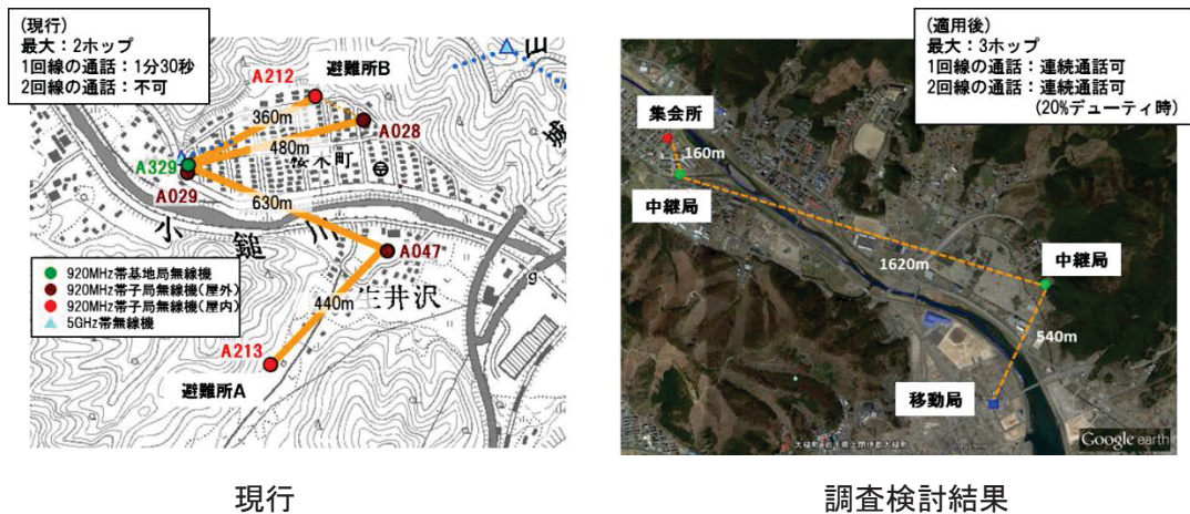
図 7-1 本調査検討会で用いた 920MHz 帯無線センサーネットワークシステムの構成
