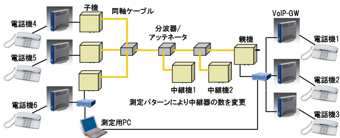
図 4-1 ラボ内試験の接続系統
