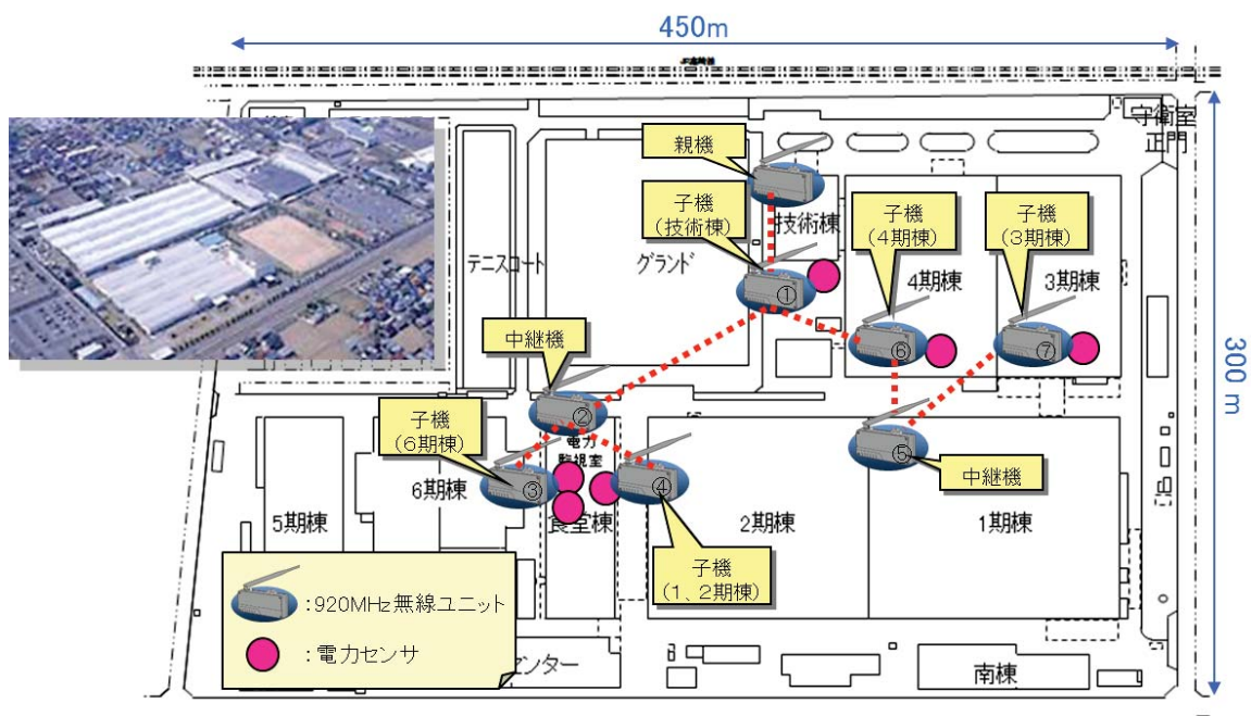
図 2-7 工場での導入事例
