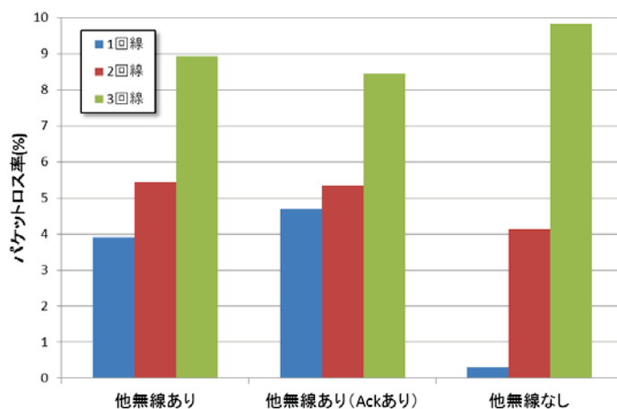
図 6-7 20mW 無線局からの被干渉 (パケットロス率)
