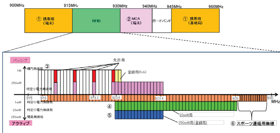
図 6-3 900MHz-960MHz 周波数使用無線システム
