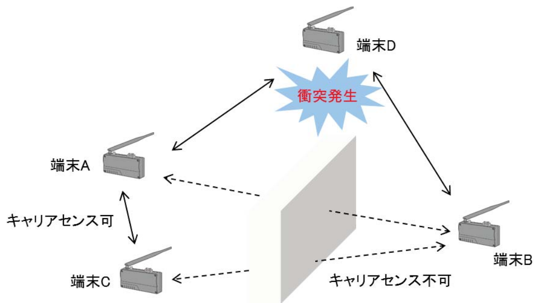
図 付 5-1 隠れ端末問題
