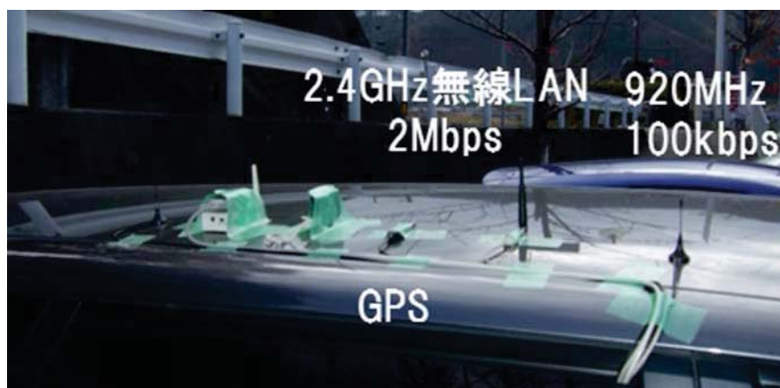
図 付 3-2 乗用車のルーフに固定した受信機の様子
