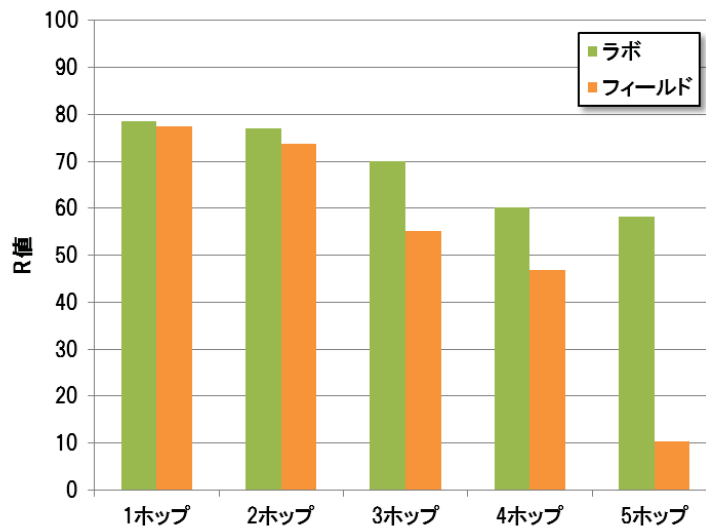
図 5-8 1 回線の Ack 無
