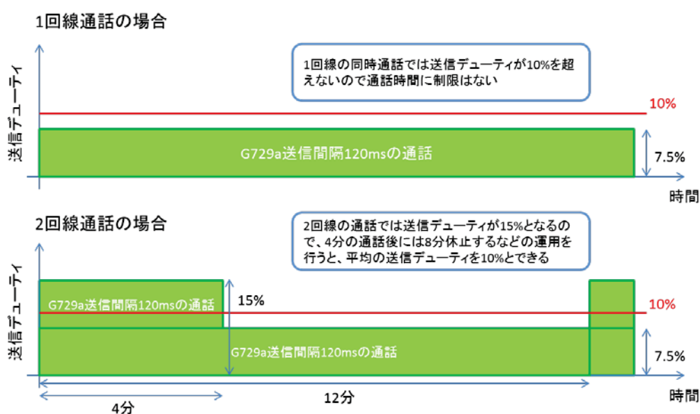
図 4-16 通話回線数と送信デューティの関係
