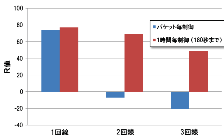
図 4-15 2 ホップ時におけるデューティ制御方式の比較(180 秒まで)
