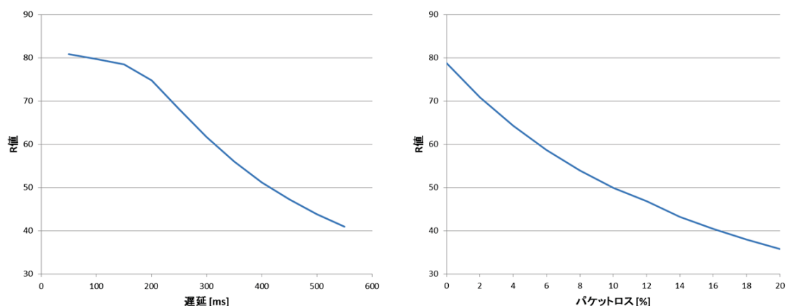
図 4-3 遅延及びパケットロスと R 値の関係
