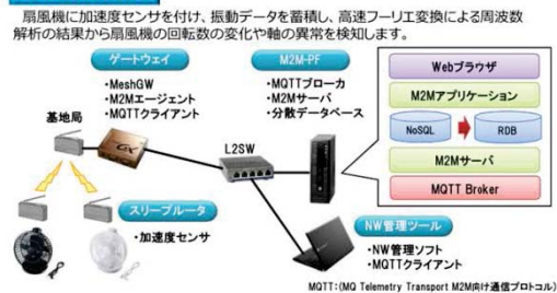
図 付 7- 4 構造物モニタリングデモのパネル
