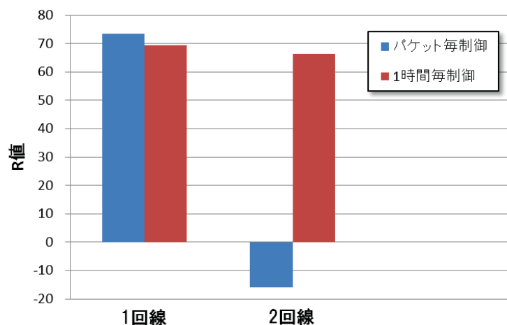
図 5-13 2 ホップの測定結果(3 分間)
