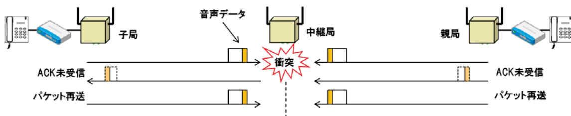
図 3-2 隠れ端末による衝突とパケット再送
