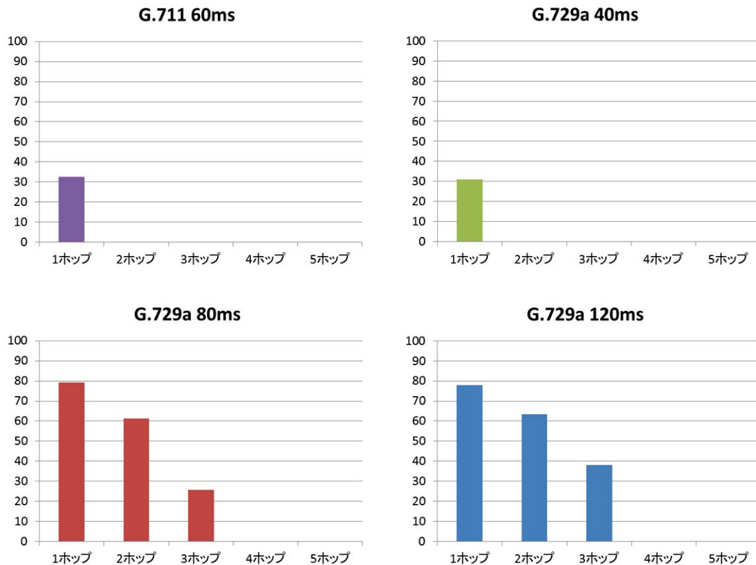
図 4-5 同時通話 2 回線の場合の各コーデックの R 値
