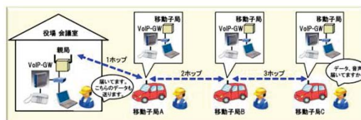
図 付 7- 3 音声データ伝送デモのパネル
