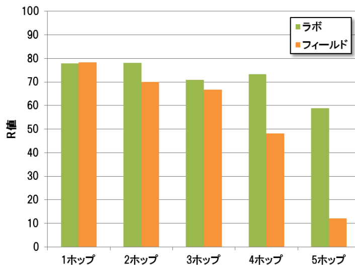
図 5-9 1 回線の Ack 有
