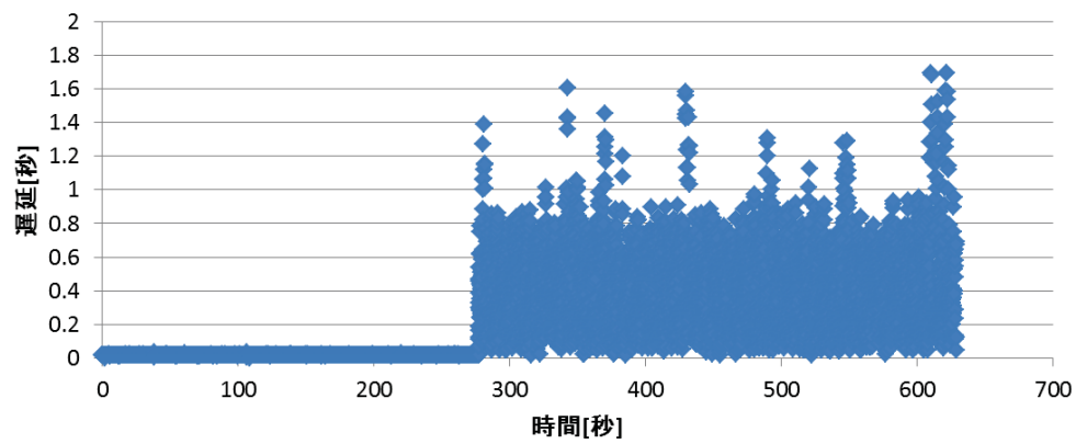
図 4-13 1 時間毎制御方式の遅延の時間変化
