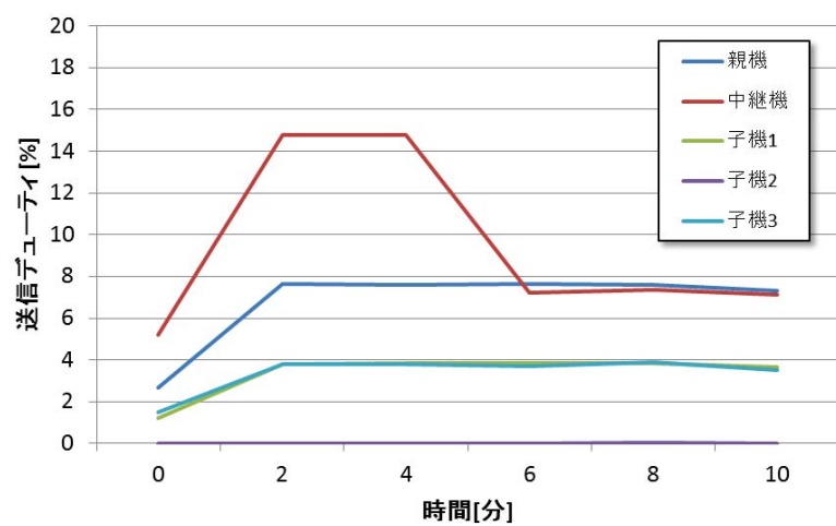
図 4-14 1 時間毎制御方式のデューティの時間変化
