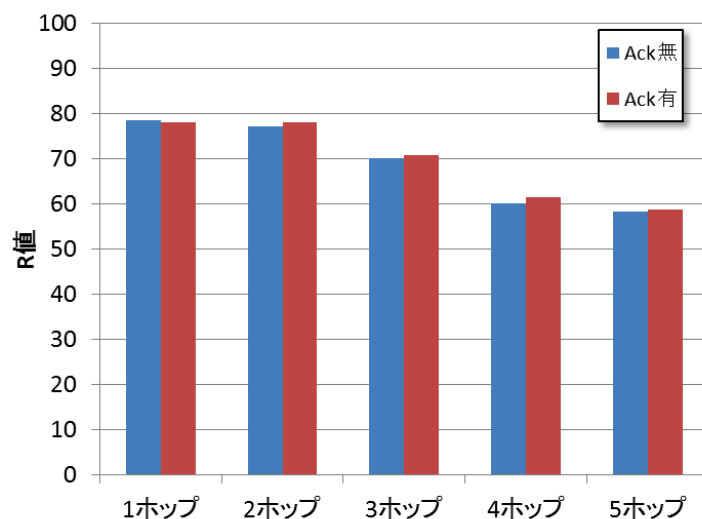
図 4-7 同時通話 1 回線の時のホップ数と R 値の関係
