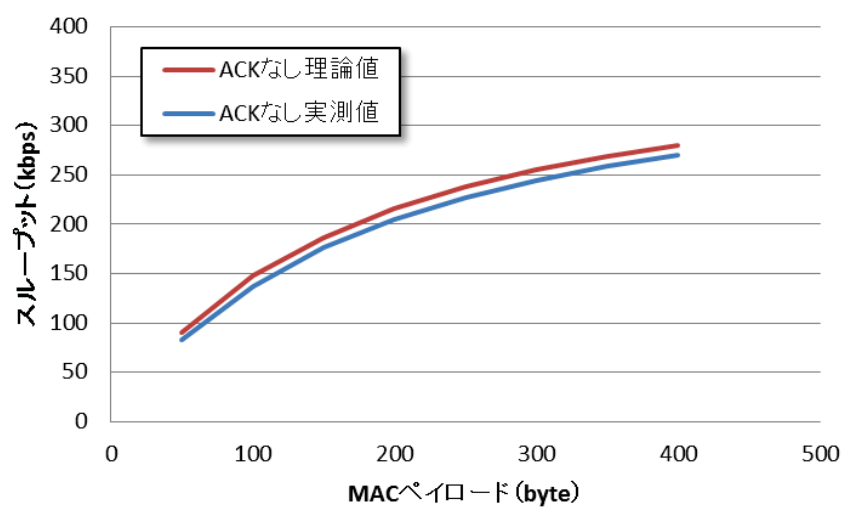
図 付 6- 1 送信ペイロード長とスループットの関係
