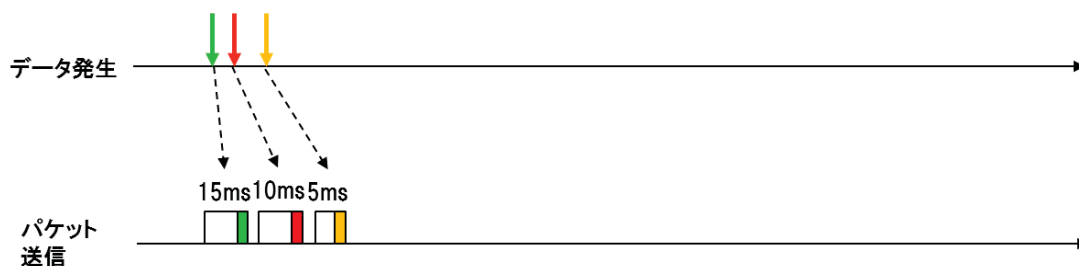
図 3-4 1 時間毎に行うデューティ制御
