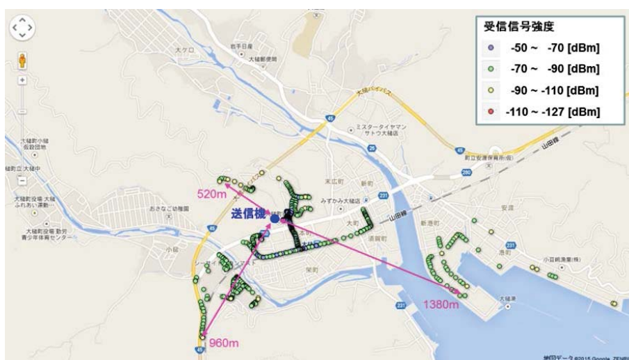
図 付 3- 5 2.4GHz 帯無線装置の受信信号強度
