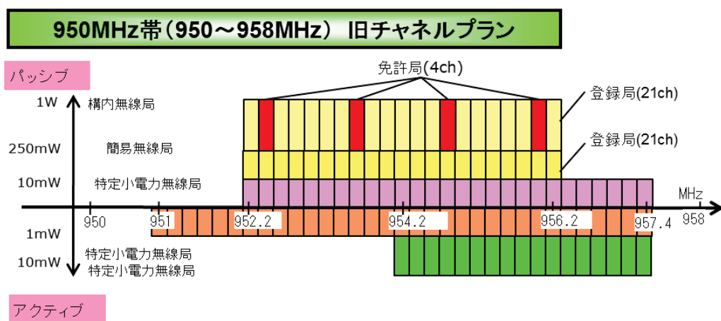
図 2-5 950MHz 帯における旧チャネルプラン
