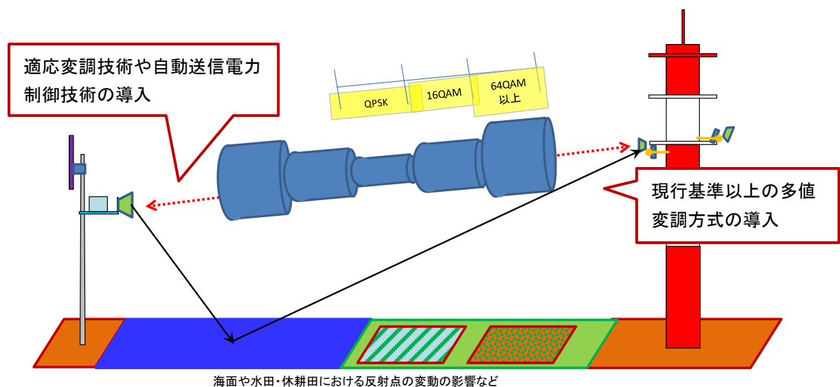
図2-6 多値変調方式及び適応変調技術等の導入時の運用イメージ
