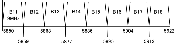
図 1-7 チャンネル配置
