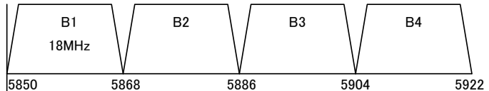
【周波数の配置と隣接チャンネル、同一チャンネルの配置】
