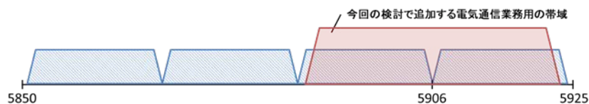
図 3-1 電気通信業務用システムの導入例 (5.8GHz 帯)
