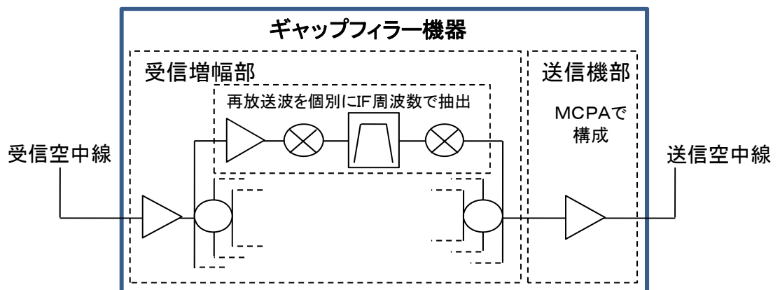
図15 ギャップフィルターの概略構成
