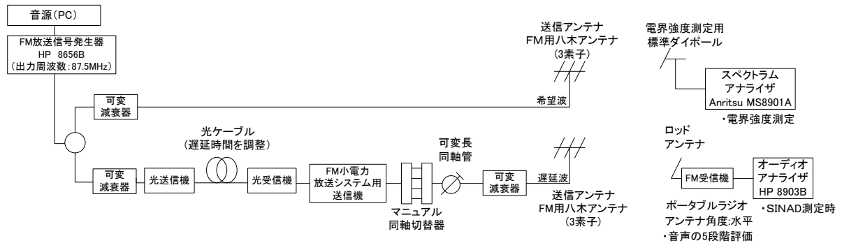
図 2 測定系統図
