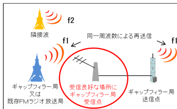
図１０ 安定した受信場所確保の例
