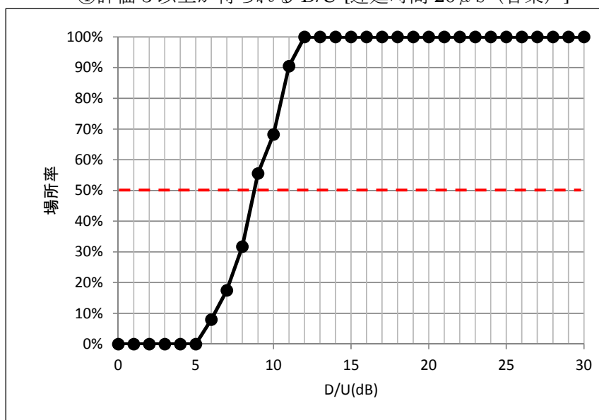
④評価 3 以上が得られる D/U [遅延時間 20\mu\text{s} (音楽) ]
