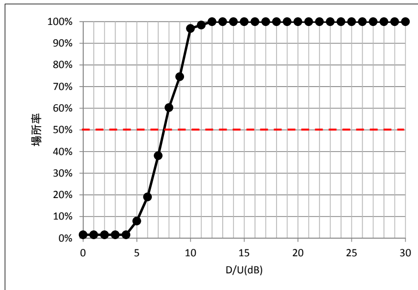
④評価 3 以上が得られる D/U [遅延時間 10\mu\text{s} (トーン信号)]
