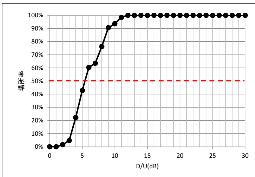
③評価 3 以上が得られる D/U [遅延時間 10\mu\text{s} (音楽) ]
