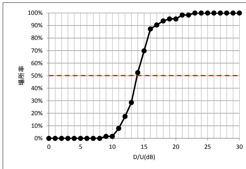
④評価 3 以上が得られる D/U [遅延時間 20\mu\text{s} (トーン信号)]
