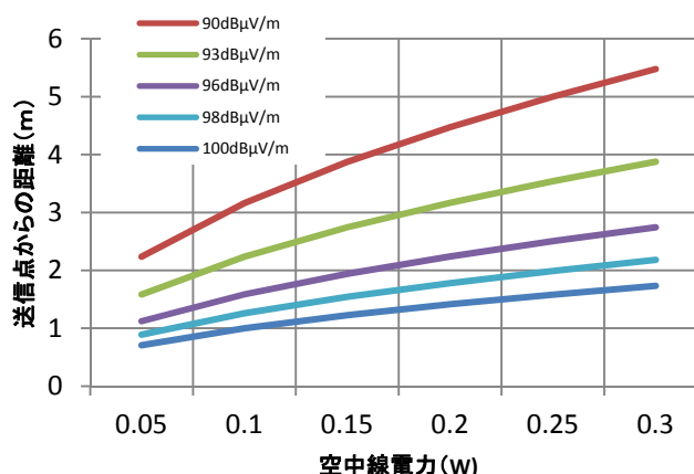
図13 ギャップフィラーの近傍電界強度(試算)
