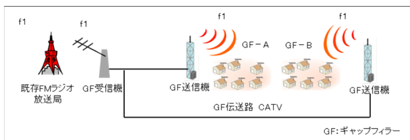
図 6 CATV網（ダークファイバー）を使用しギャップファイラー同士の放送区域の重なりがある場合（双方に関わる条件がある）
