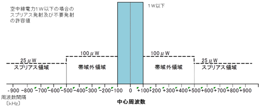
図 1 8 空中線電力 1 W以下のスプリアス発射又は不要発射の強度
