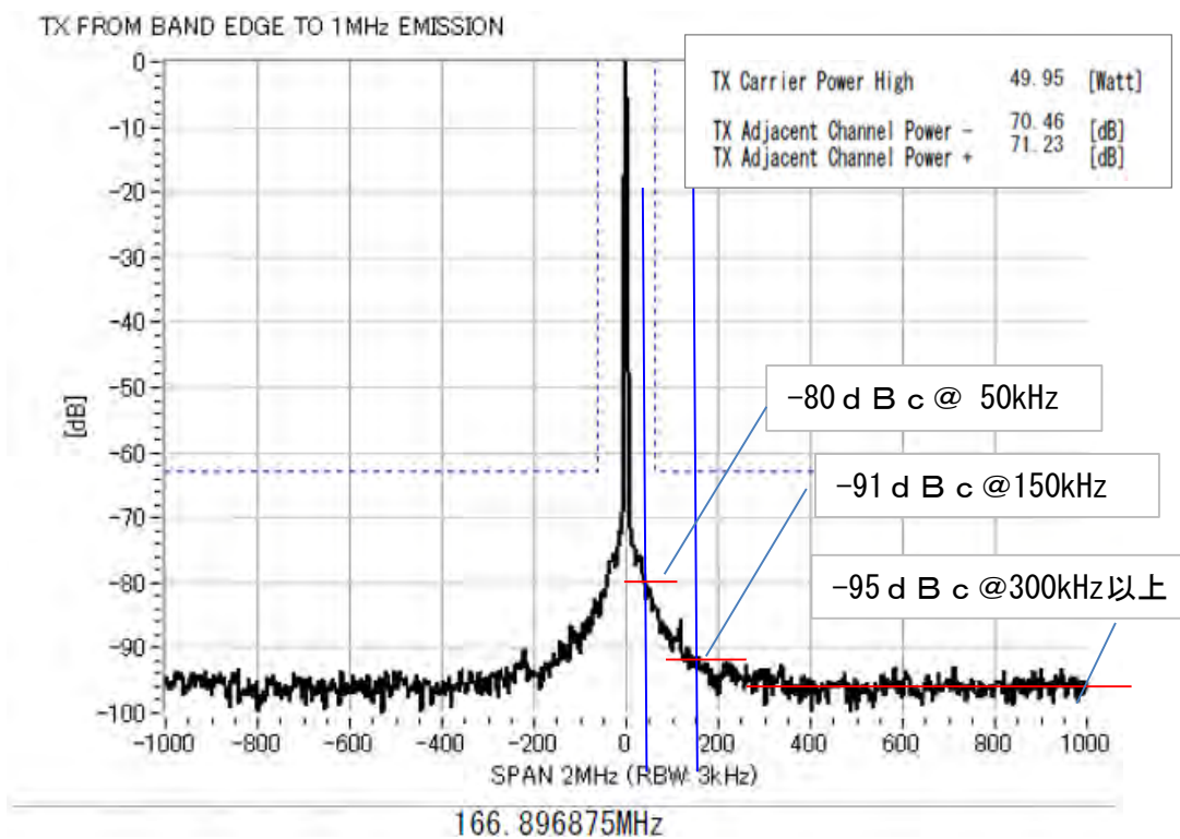
図 1 7 移動局（中継車）（50W）のスペクトル波形（サンプルデータ）
