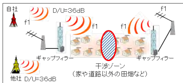
図7 ギャップフィラー間の放送区域に発生する干渉エリアの例
