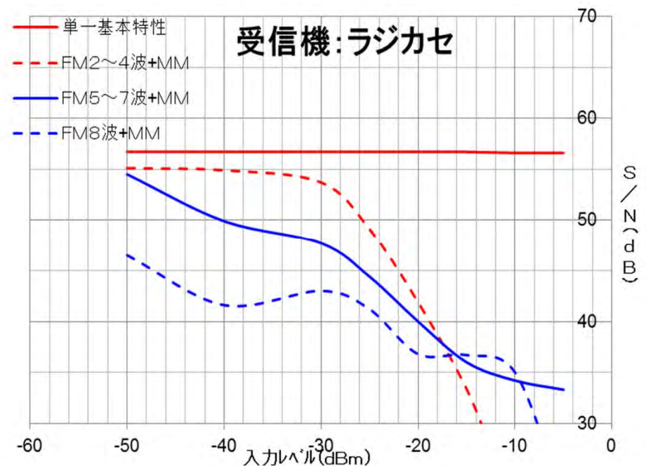
276 FM放送波2～8波+MM受信時の特性
