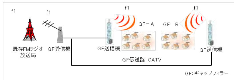
図 6 CATV網（ダークファイバー）を使用し ギャップフィラー同士の放送区域の重なりがある場合 （双方に関わる条件がある）
