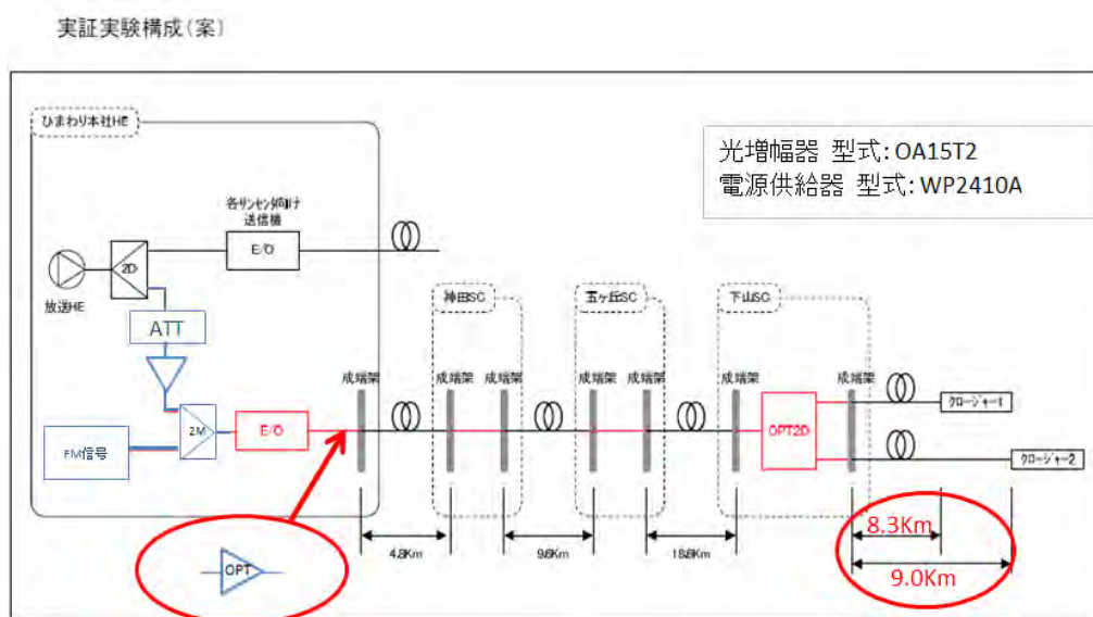
図 5 送信点 1 と送信点 2 のクロージャまでの光ケーブル長
